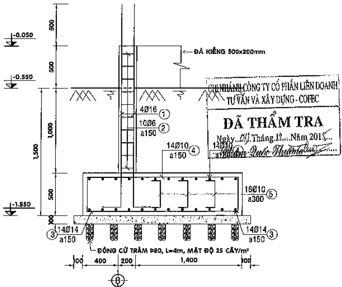
MẶT CẮT 3-3 - TL 1/25
