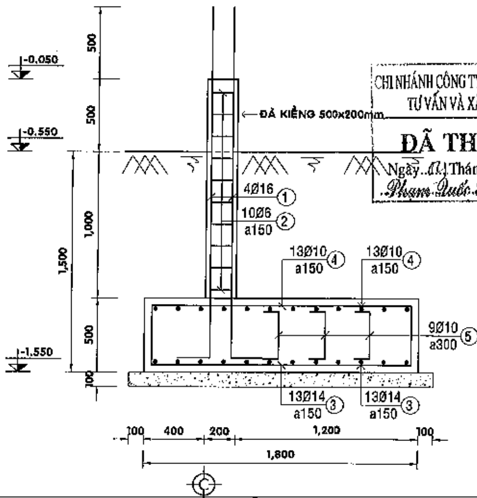
MẶT CẮT 4-4 - TL 1/25
