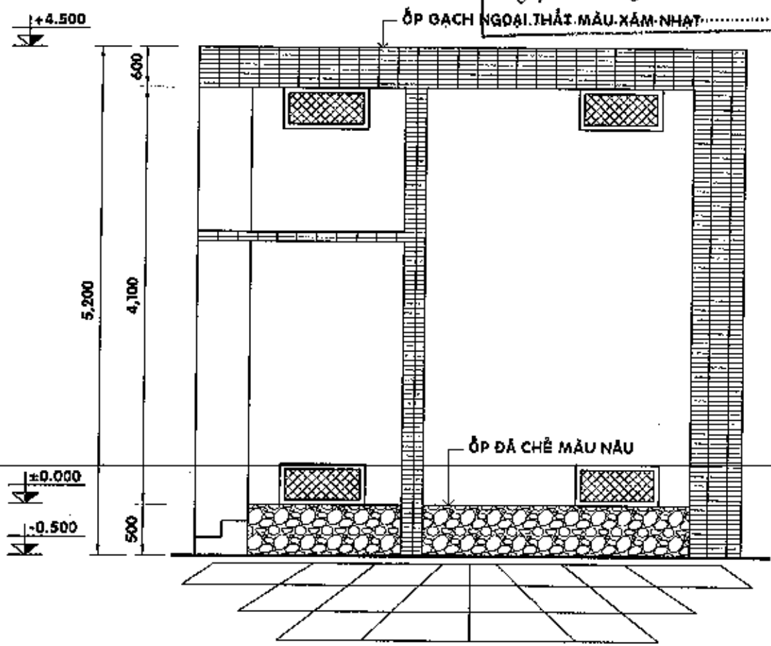
MẶT ĐỨNG TRỤC A-B - TL 1/50
