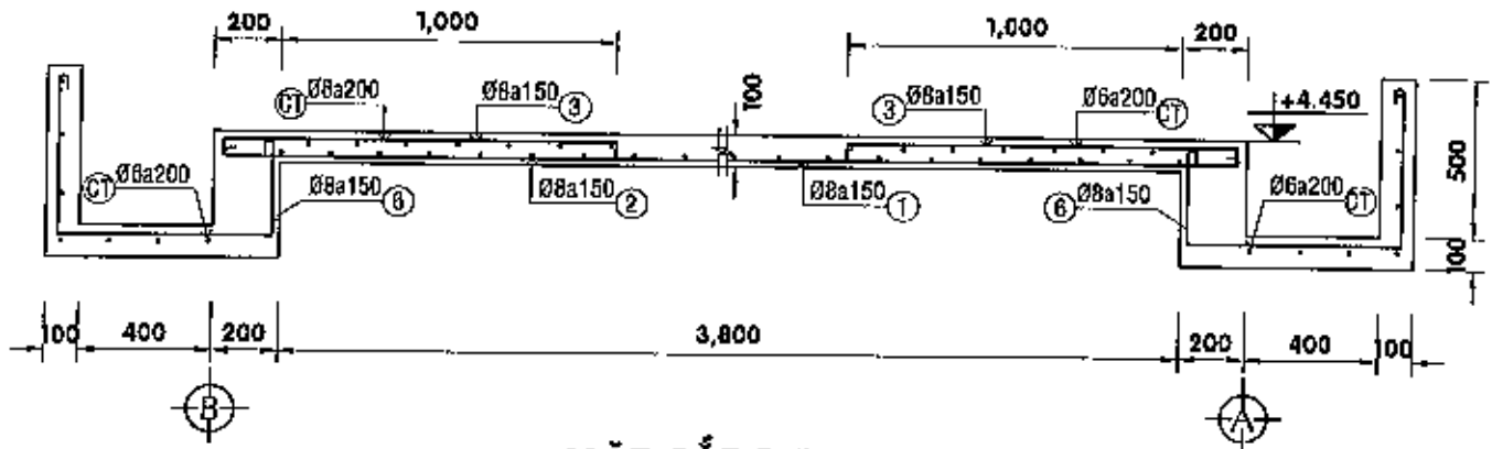
MẶT CẮT B-B - TL 1/25
