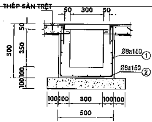
MƯỜNG HẠ THỂ - TL 1/20
