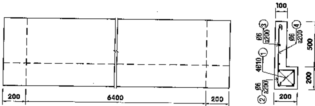
CỘT THÉP LAM CHE NẮNG - TL 1/20
