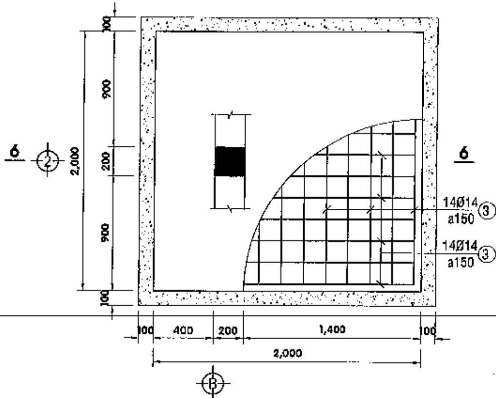
KẾT CẤU MÓNG M2 - TL 1/25 (LOẠI 3: KÍCH THƯỚC 1.8mx1.8m)
