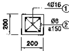
CỘT THÉP CỘT - TL 1/20
