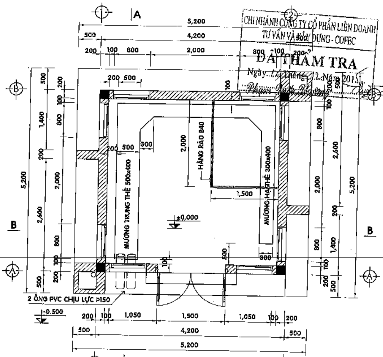
MẶT BẰNG TRẠM - TL 1/50
