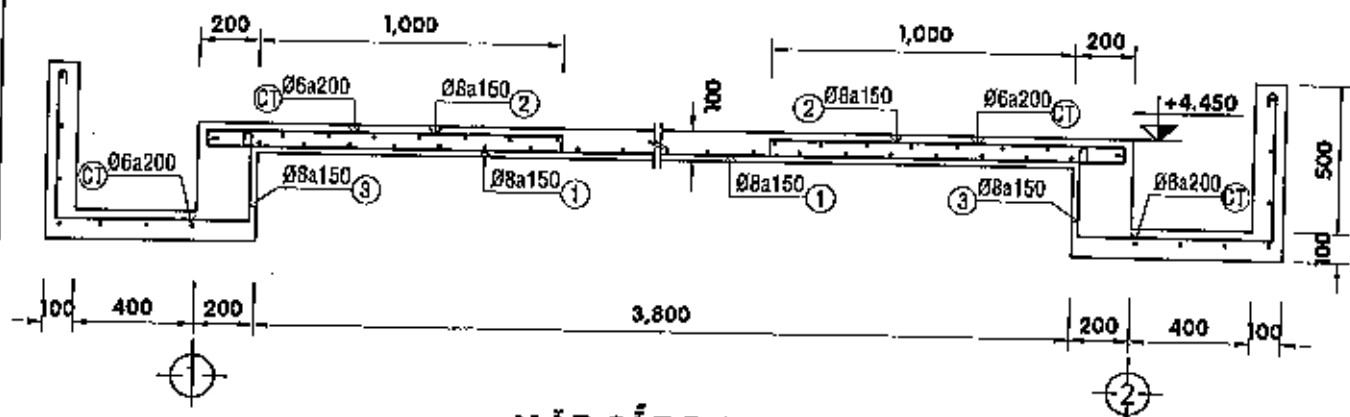
MẶT CẮT B-B - TL 1/25
