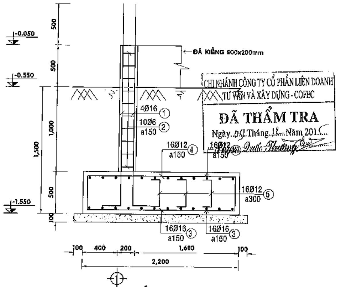
MẶT CẮT 2-2 - TL 1/25
