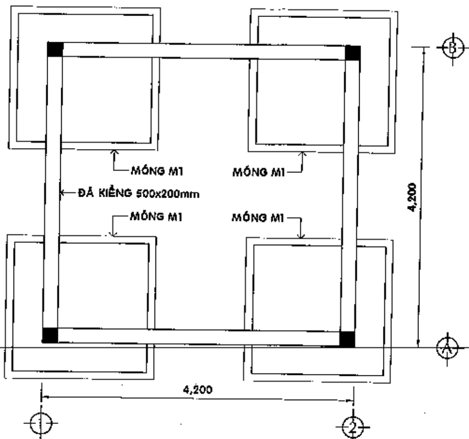
MẶT BẰNG BỐ TRÍ MÓNG - TL 1/50
