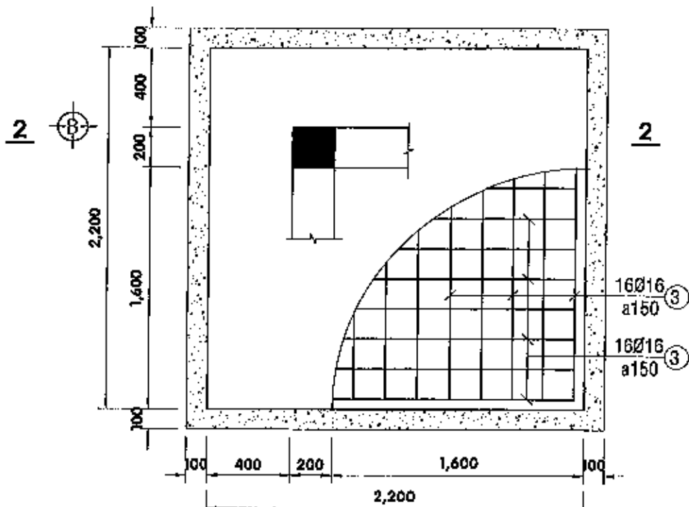
KẾT CẤU MÓNG M1 - TL 1/25 (LOẠI 2: KÍCH THƯỚC 2.2mx2.2m)
