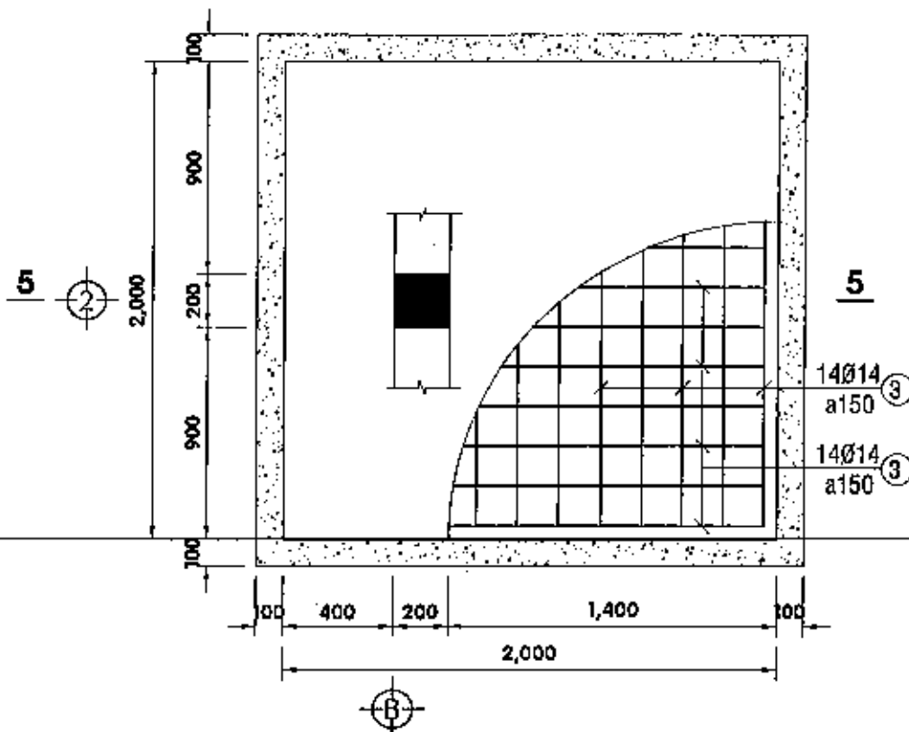
KẾT CẤU MÓNG M2 - TL 1/25 (LOẠI 2: KÍCH THƯỚC 2.0mx2.0m)
