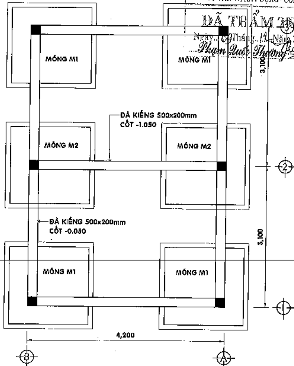
MẶT BẰNG BỐ TRÍ MÓNG - TL 1/50
