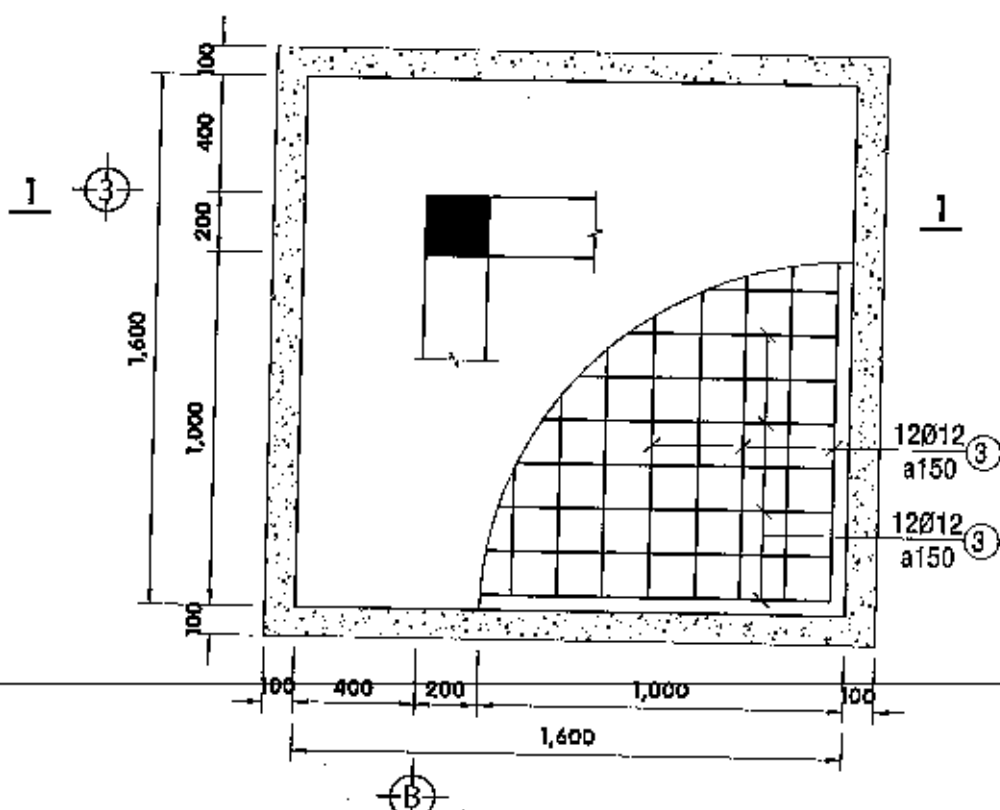
KẾT CẤU MÓNG M1 - TL 1/25 (LOẠI 1: KÍCH THƯỚC 1.6mx1.6m)
