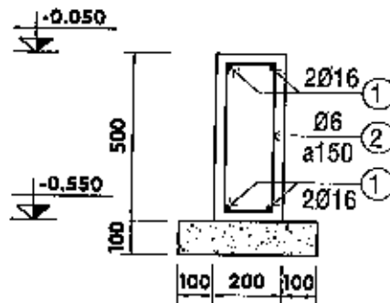
CỘT THÉP ĐÀ KIỀNG - TL 1/20
