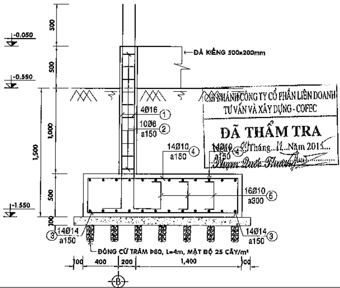
MẶT CẮT 6-6 - TL 1/25
