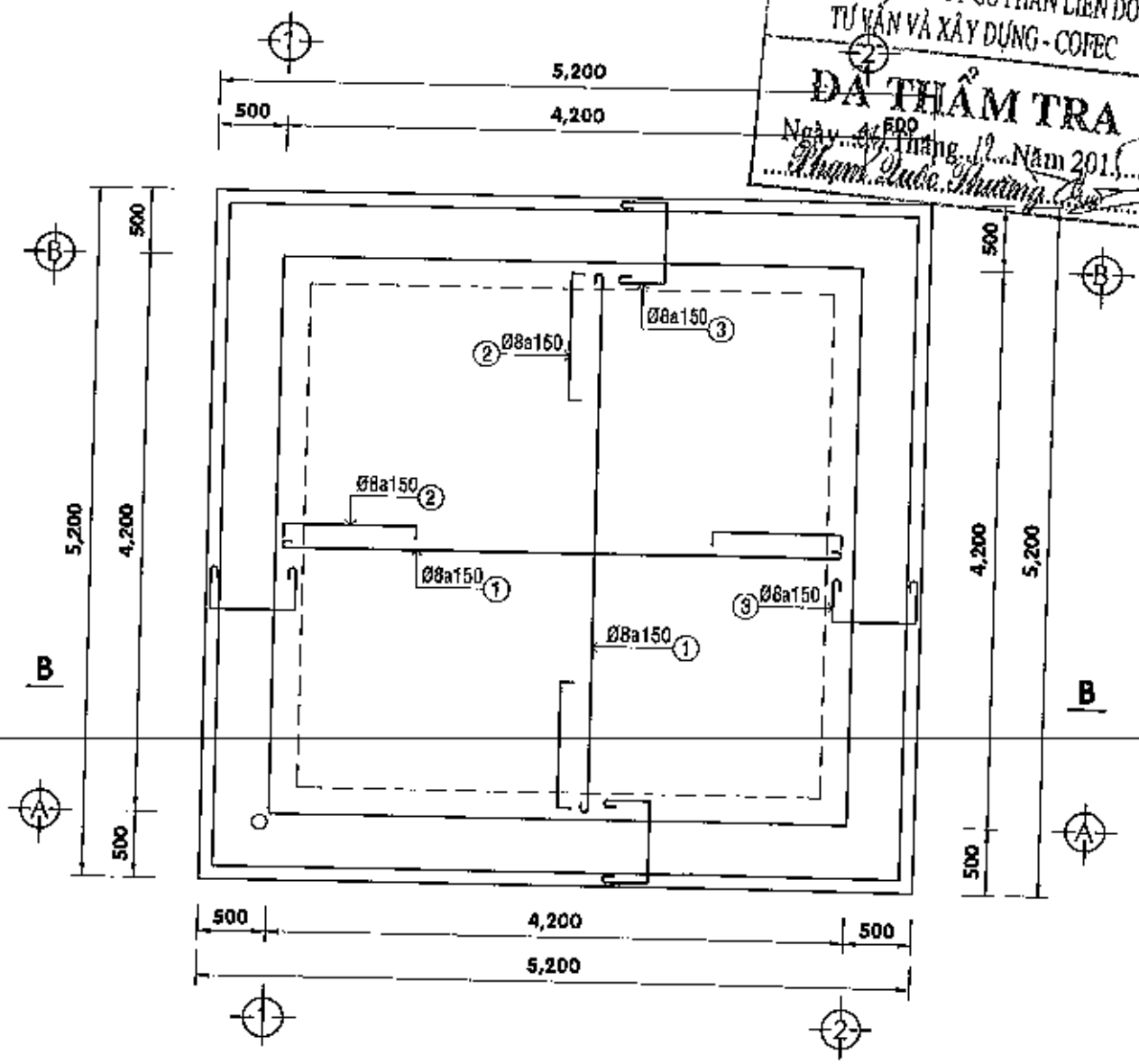
MẶT BẰNG THÉP SÀN MÁI - TỈ 1/50
