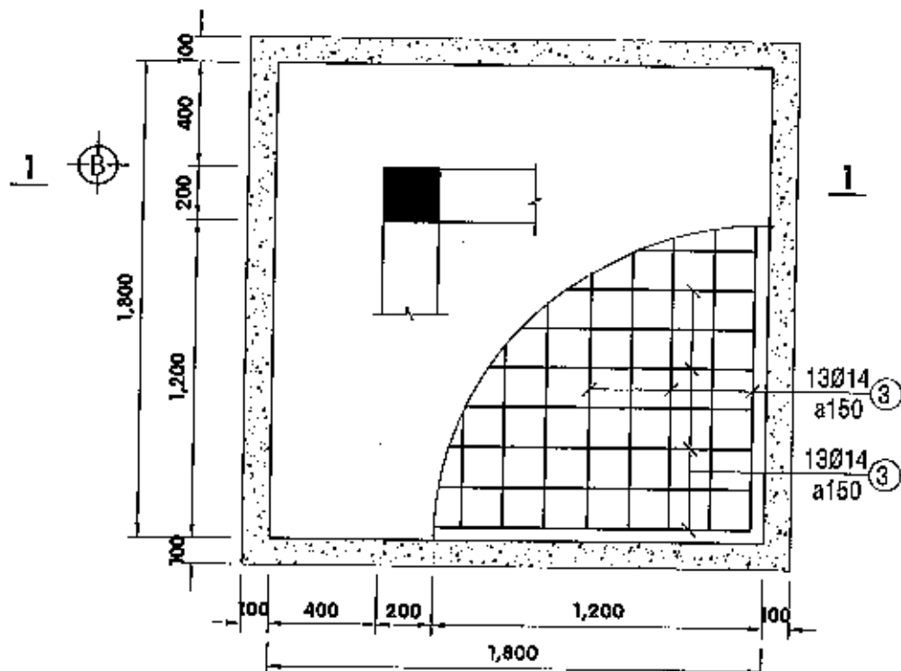
KẾT CẤU MÓNG M1 - TL 1/25 (LOẠI 1: KÍCH THƯỚC 1.8mx1.8m)
