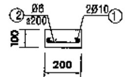
CỘT THÉP LANH TÔ THÔNG GIÓ - TL 1/20
