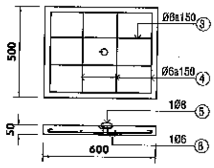
MƯỜNG TRUNG THỂ - TL 1/20
