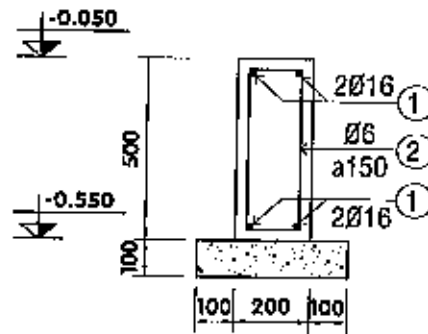
CỐT THÉP ĐÀ KIỀNG - TL 1/20
