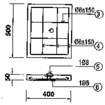
MƯỜNG HẠ THỂ - TL 1/20
