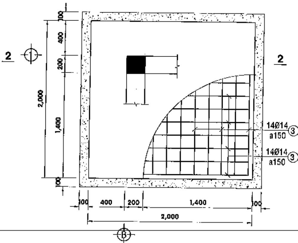
KẾT CẤU MÓNG M1 - TL 1/25 (LOẠI 2: KÍCH THƯỚC 2.0m x 2.0m)
