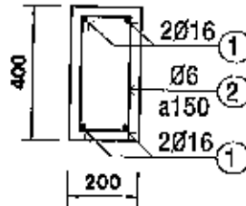
CỘT THÉP DẦM MÃI - TL 1/20
