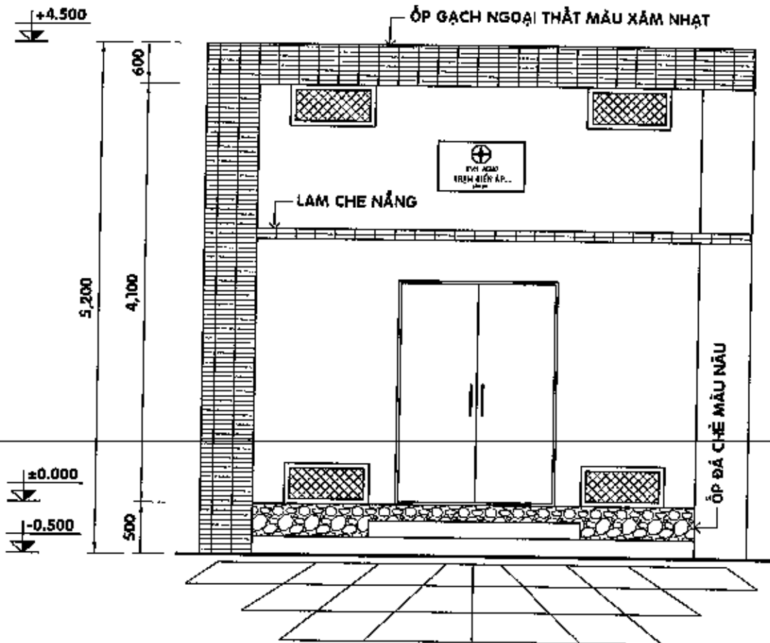
MẶT ĐỨNG TRỰC 1-2 - TL 1/50
