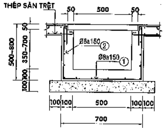
MƯỜNG TRUNG THỂ - TL 1/20
