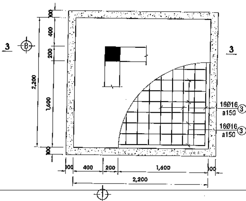
KẾT CẤU MÓNG M1 - TL 1/25 (LOẠI 3: KÍCH THƯỚC 2.2m x 2.2m)
