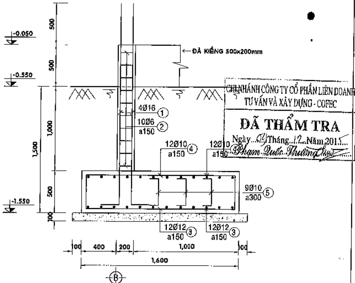
MẶT CẮT 1-1 - TL 1/25
