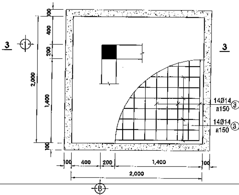
KẾT CẤU MÓNG M1 - TL 1/25 (LOẠI 3: KÍCH THƯỚC 2.0mx2.0m)
