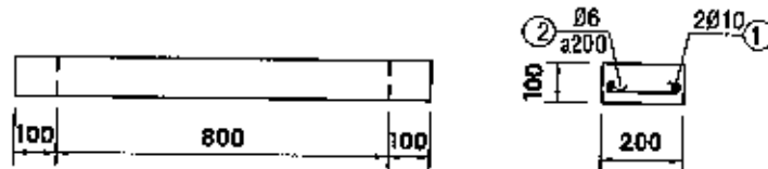
CỘT THÉP LANH TỔ THÔNG GIÓ - TL 1/20
