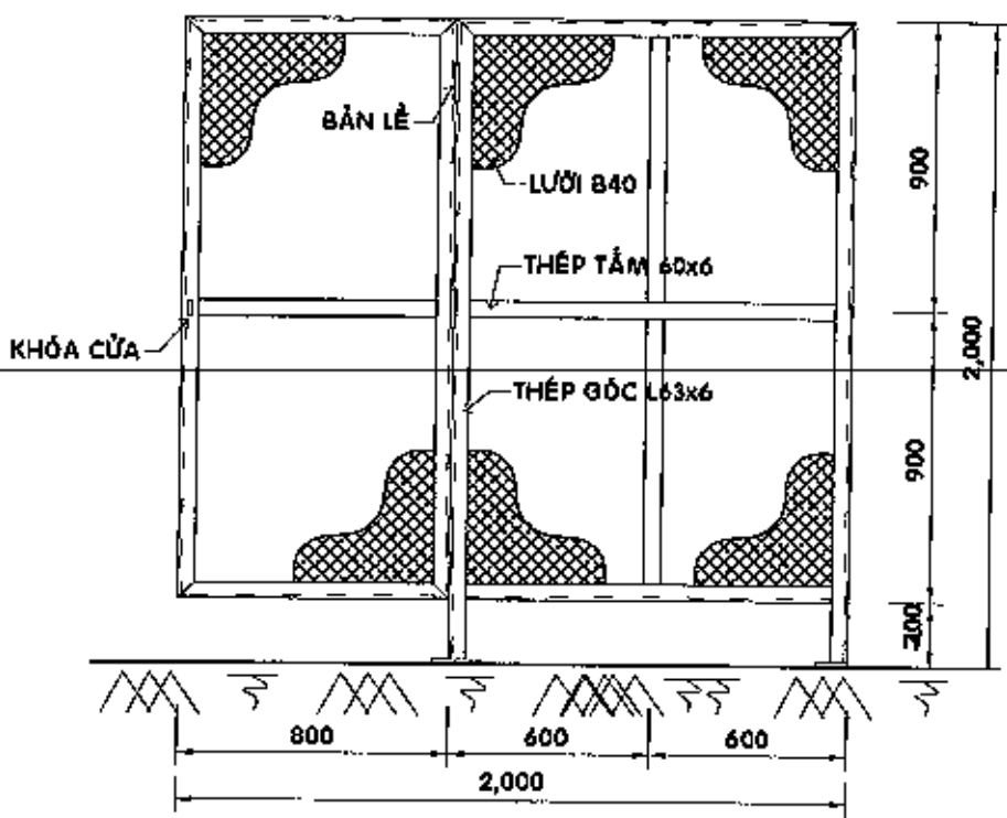
CHI TIẾT HÀNG RÀO LƯỚI B40 - TL 1/25
