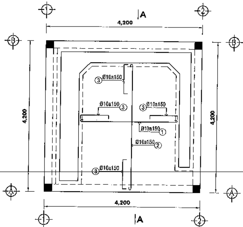
MẶT BẰNG THÉP SÀN TRỆT - TL 1/50
