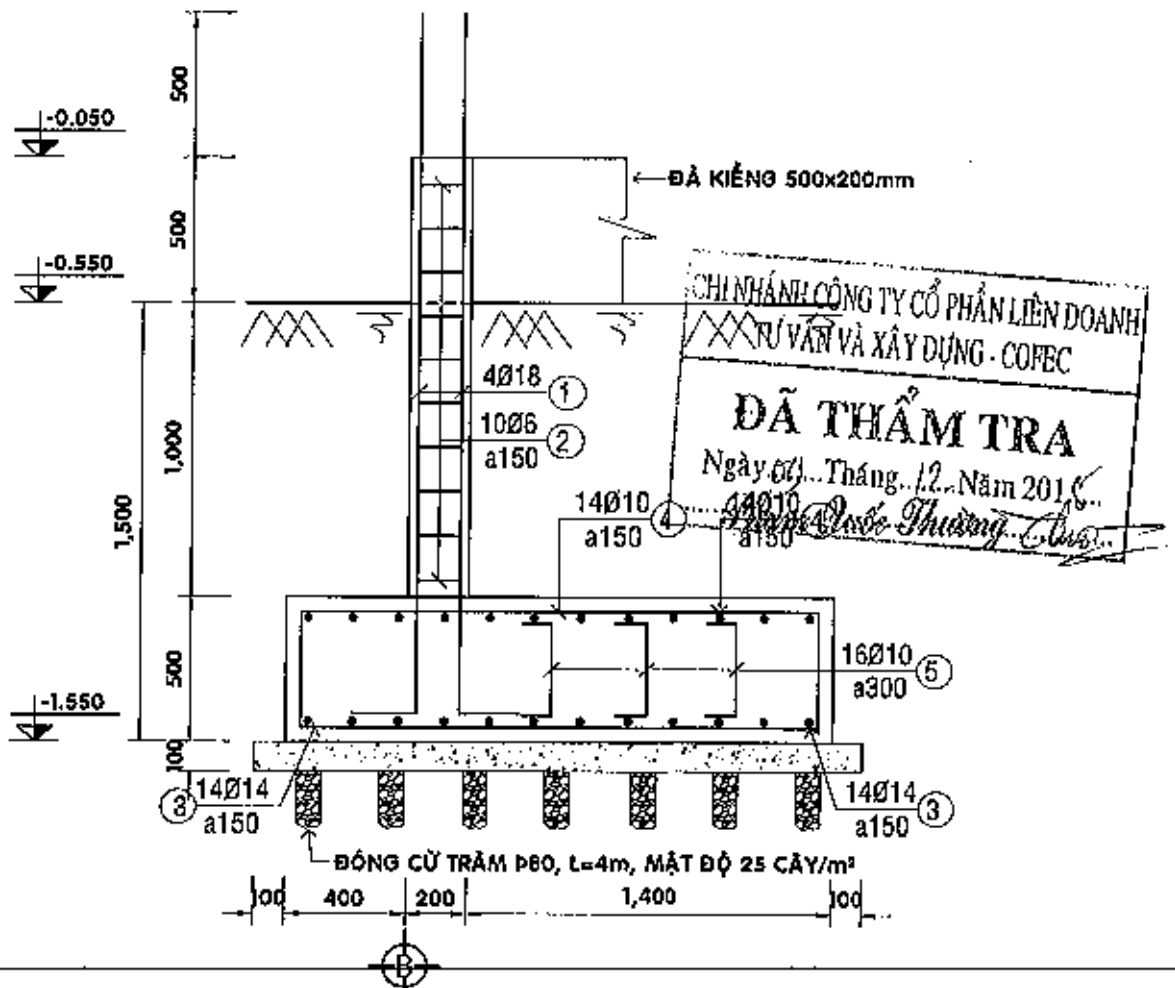
MẶT CẮT 9-9 - TL 1/25
