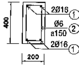
THÉP DẦM MÁI BIÊN TL 1/20
