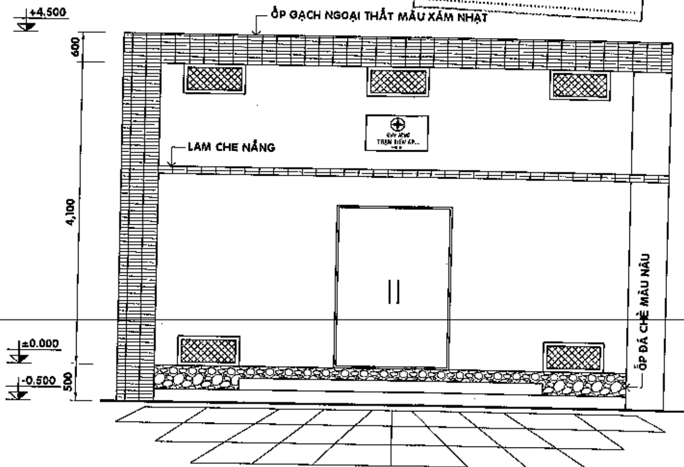
MẶT ĐỨNG TRỰC 1-3 - TL 1/50
