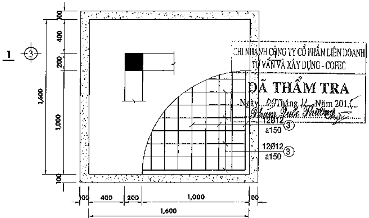
KẾT CẤU MÓNG M1 - TL 1/25 (LOẠI 1: KÍCH THƯỚC 1.6mx1.6m)
