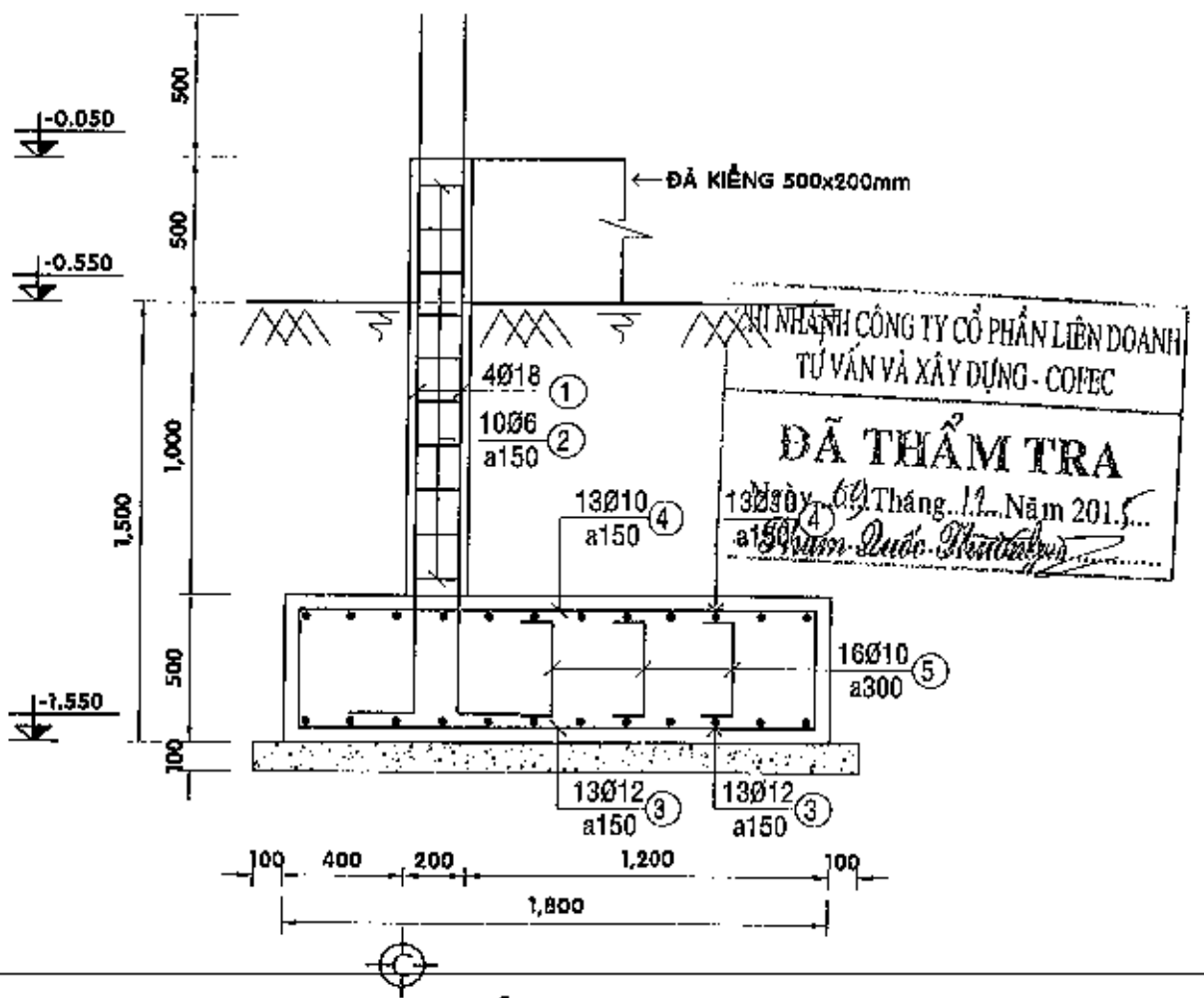
MẶT CẮT 2-2 - TL 1/25
