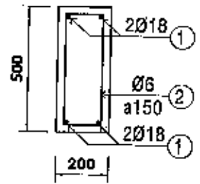
THÉP DẦM MÁI GIỮA TL 1/20
