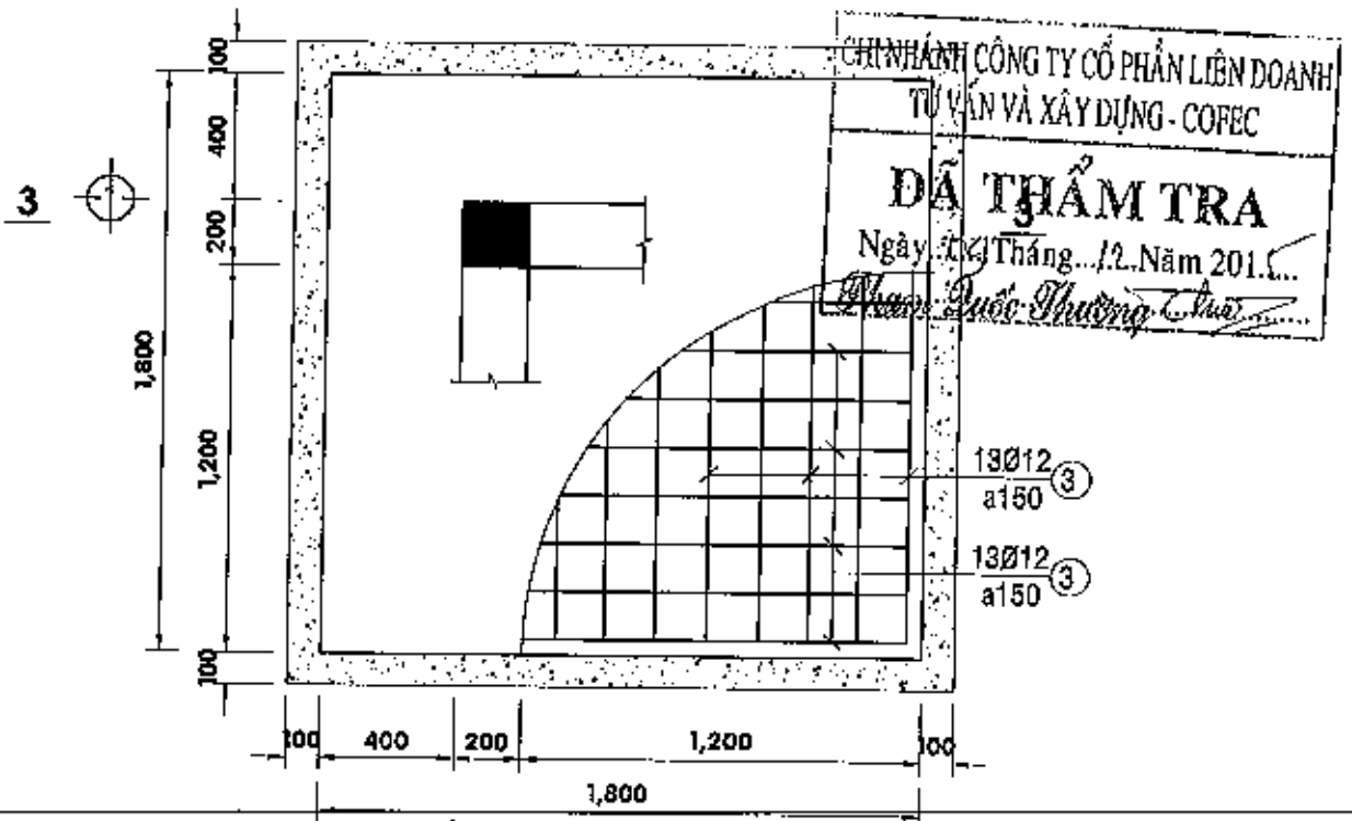
KẾT CẤU MÓNG M1 - TL 1/25 (LOẠI 3: KÍCH THƯỚC 1.8mx1.8m)
