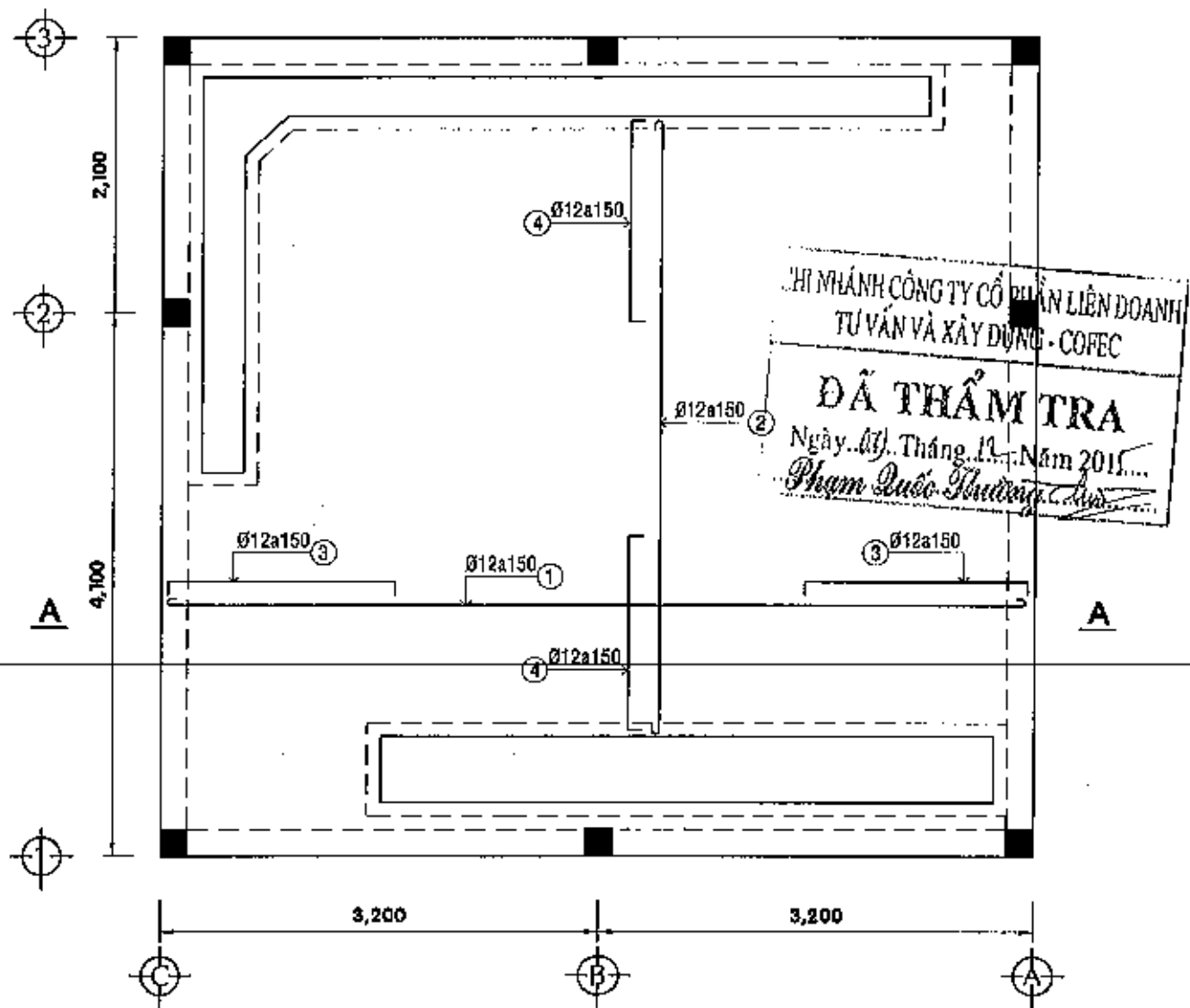
MẶT BẰNG THÉP SÀN TRỆT - TL 1/50
