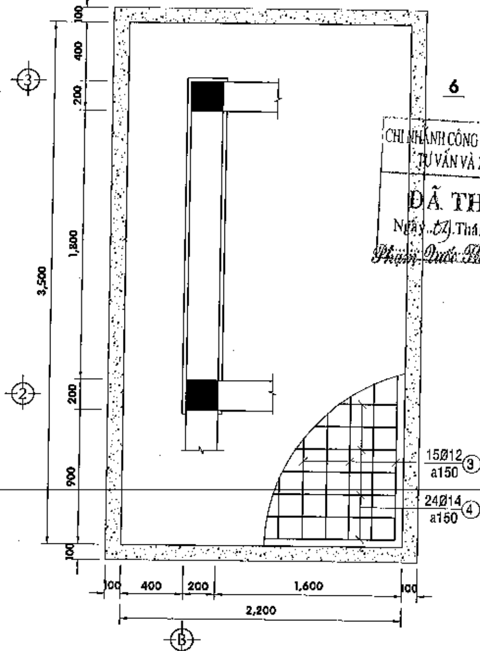
KẾT CẤU MÓNG M2 - TL 1/25 (LOẠI 3: KÍCH THƯỚC 3.5mx2.2m)
