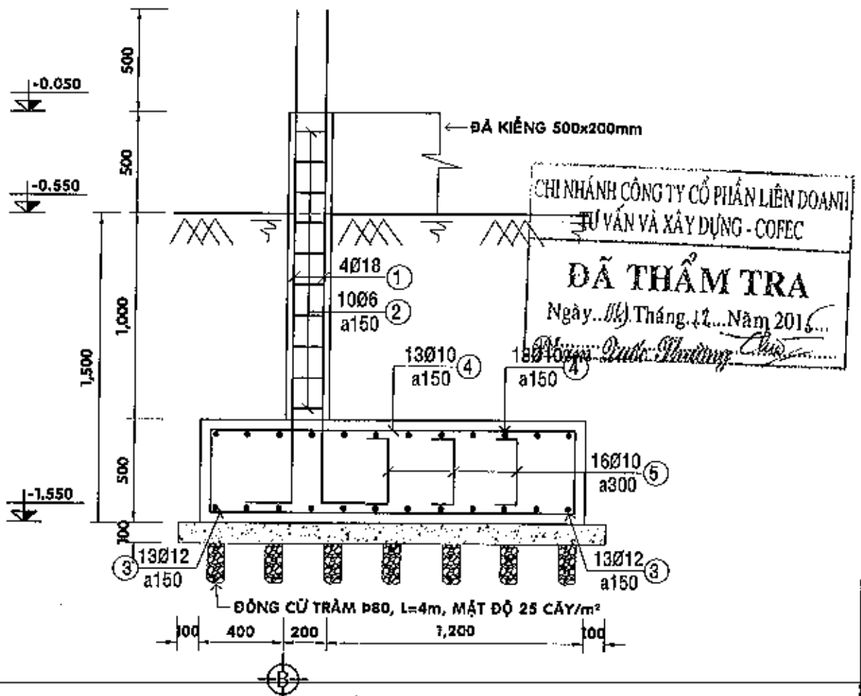
MẶT CẮT 3-3 - TL 1/25
