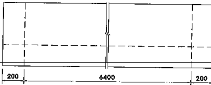
CỘT THÉP LAM CHE NẶNG - TL 1/20
