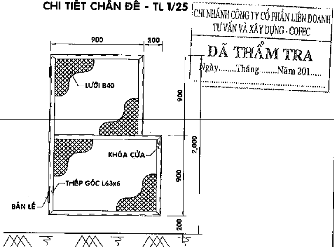
CHI TIẾT HÀNG RÀO LƯỚI B40 - TL 1/25
