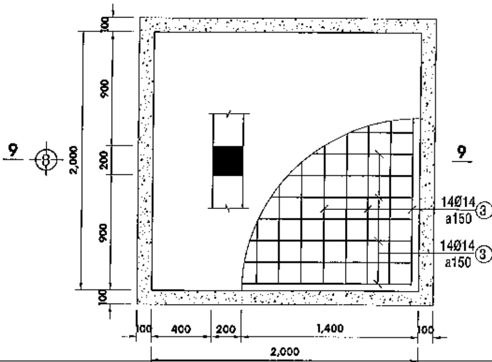
KẾT CẤU MÓNG M3 - TL 1/25 (LOẠI 3: KÍCH THƯỚC 1.8mx1.8m)
