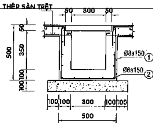
MƯNG HẠ THỂ - TL 1/20
