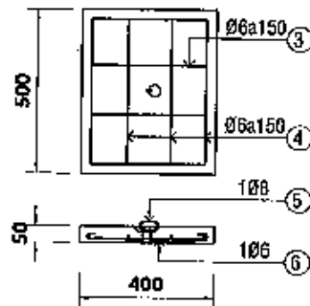
MƯNG HẠ THỂ - TL 1/20
