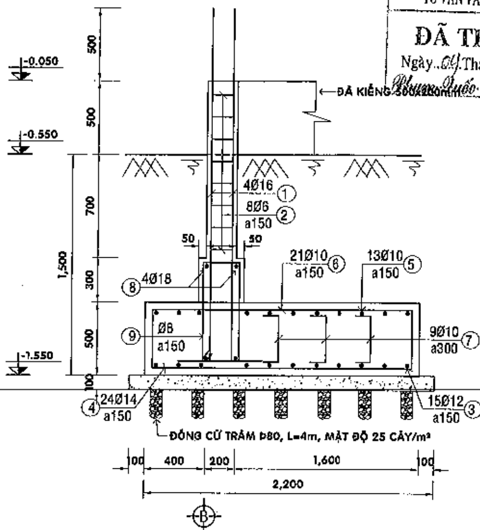
MẶT CẮT 6-6 - TL 1/25
