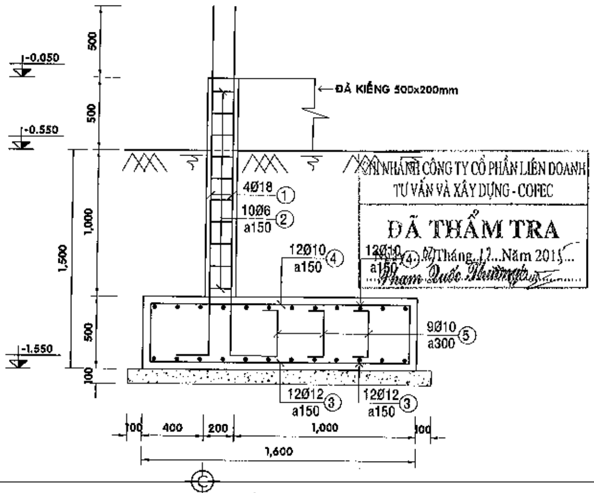
MẶT CẮT 1-1 - TL 1/25
