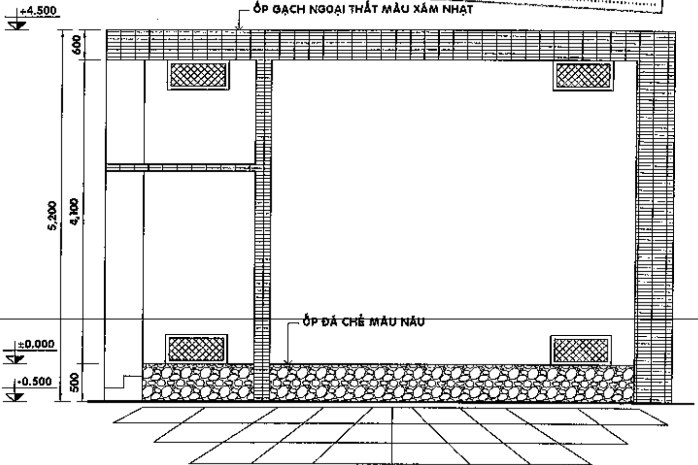
MẶT ĐỨNG TRỤC A-C - TL 1/50
