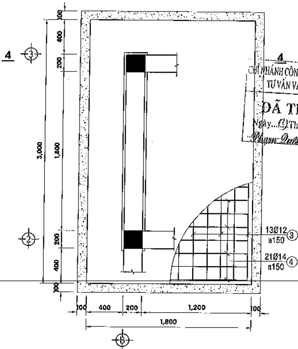
KẾT CẦU MÔNG M2 - TL 1/25 (LOẠI 1: KÍCH THƯỚC 3.0mx1.8m)
