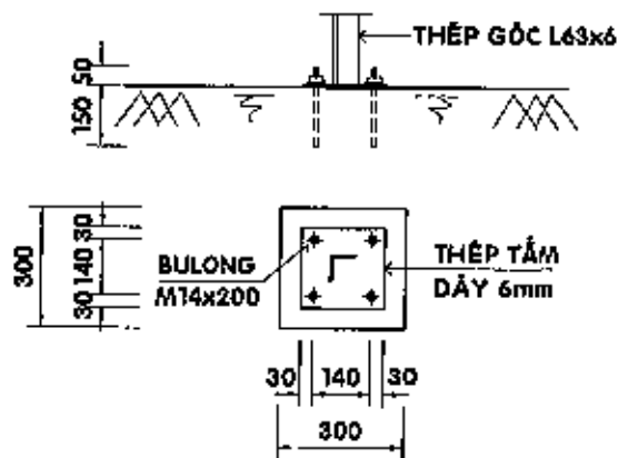
CHI TIẾT CHÂN ĐỀ - TL 1/25
