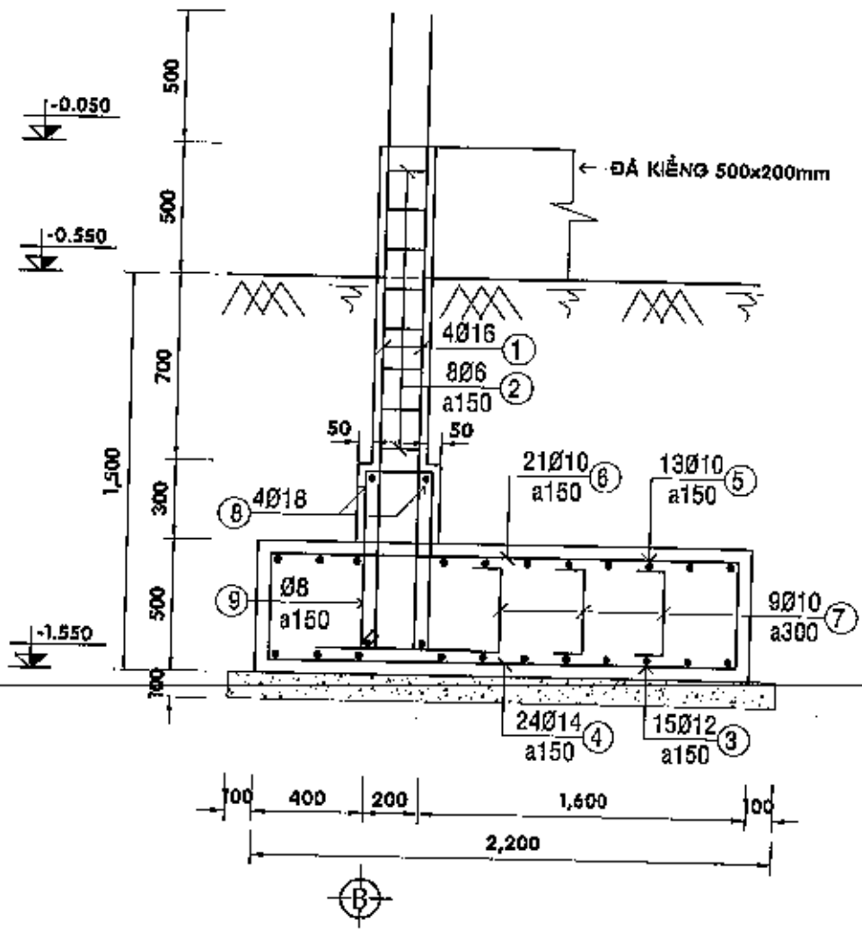
MẶT CẮT 5-5 - TỈ LỆ 1/25
