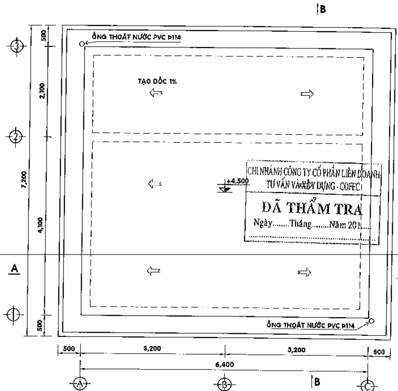
MẶT BẰNG MÁI - TL 1/50
