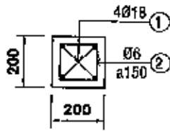
THÉP CỘT TL 1/20
