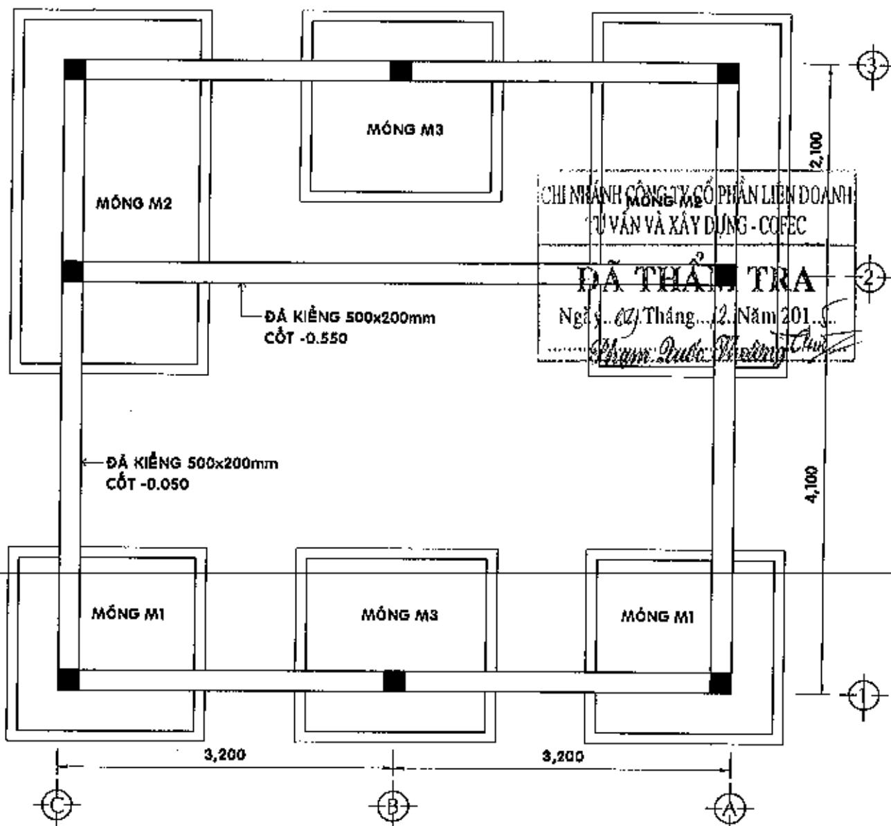
MẶT BẰNG BỐ TRÍ MÓNG - TL 1/50
