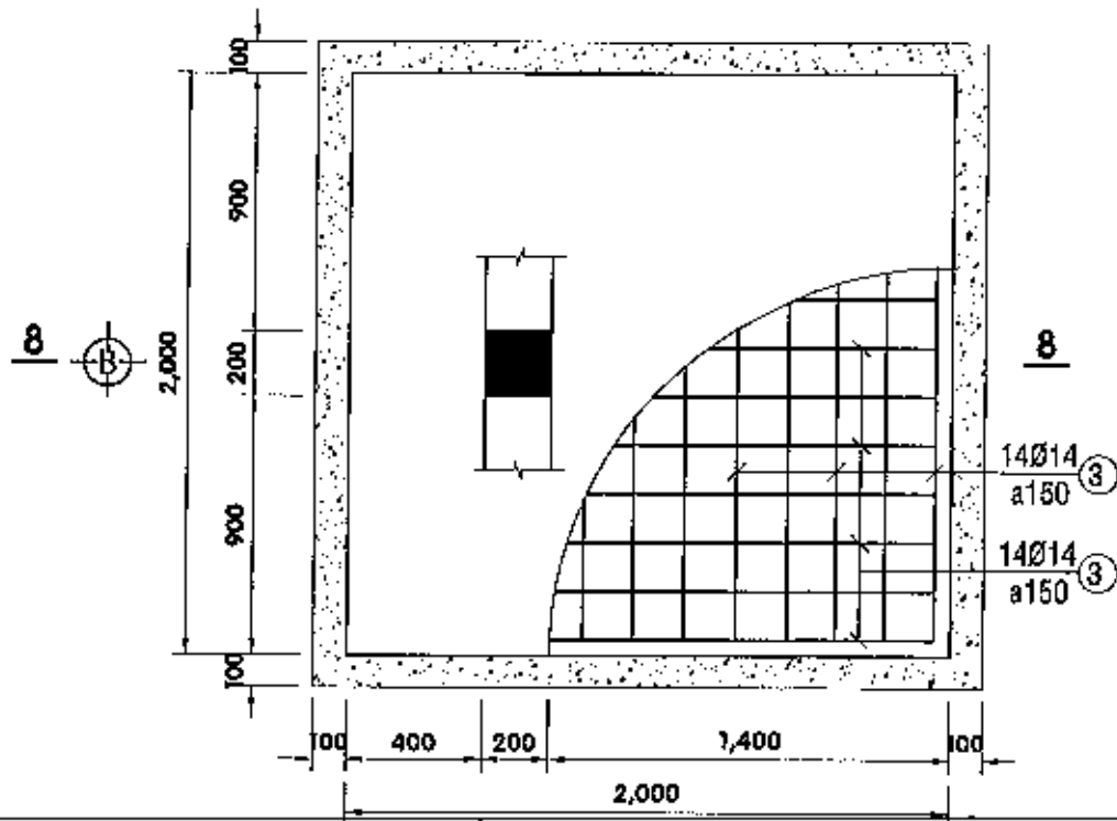
KẾT CẦU MÓNG M3 - TL 1/25 (LOẠI 2; KÍCH THƯỚC 2.0m x 2.0m)
