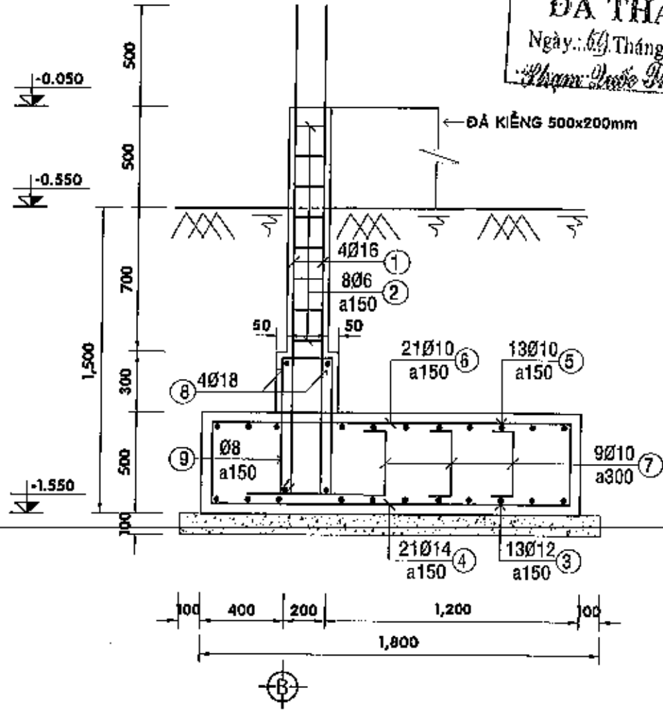
MẶT CẮT 4-4 - TL 1/25
