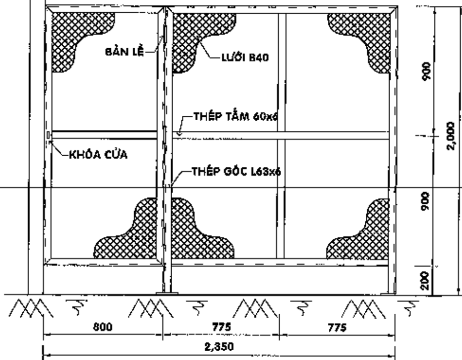
CHI TIẾT HÀNG RÀO LƯỚI B40 - TL 1/25
