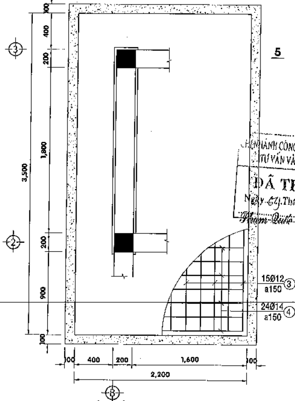
KẾT CẦU MÓNG M2 - TL 1/25 (LOẠI 2: KÍCH THƯỚC 3.5mx2.2m)
