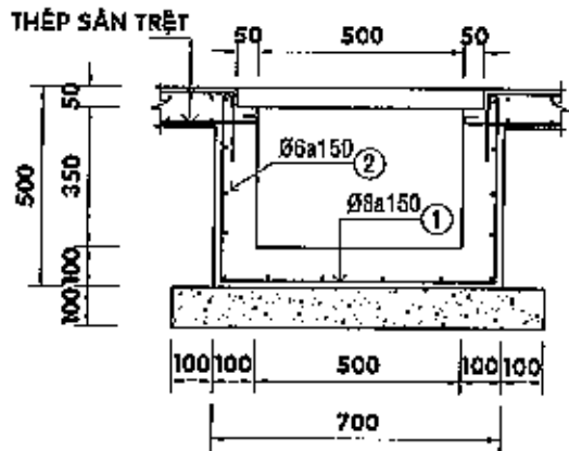
MƯNG TRUNG THỂ - TL 1/20
