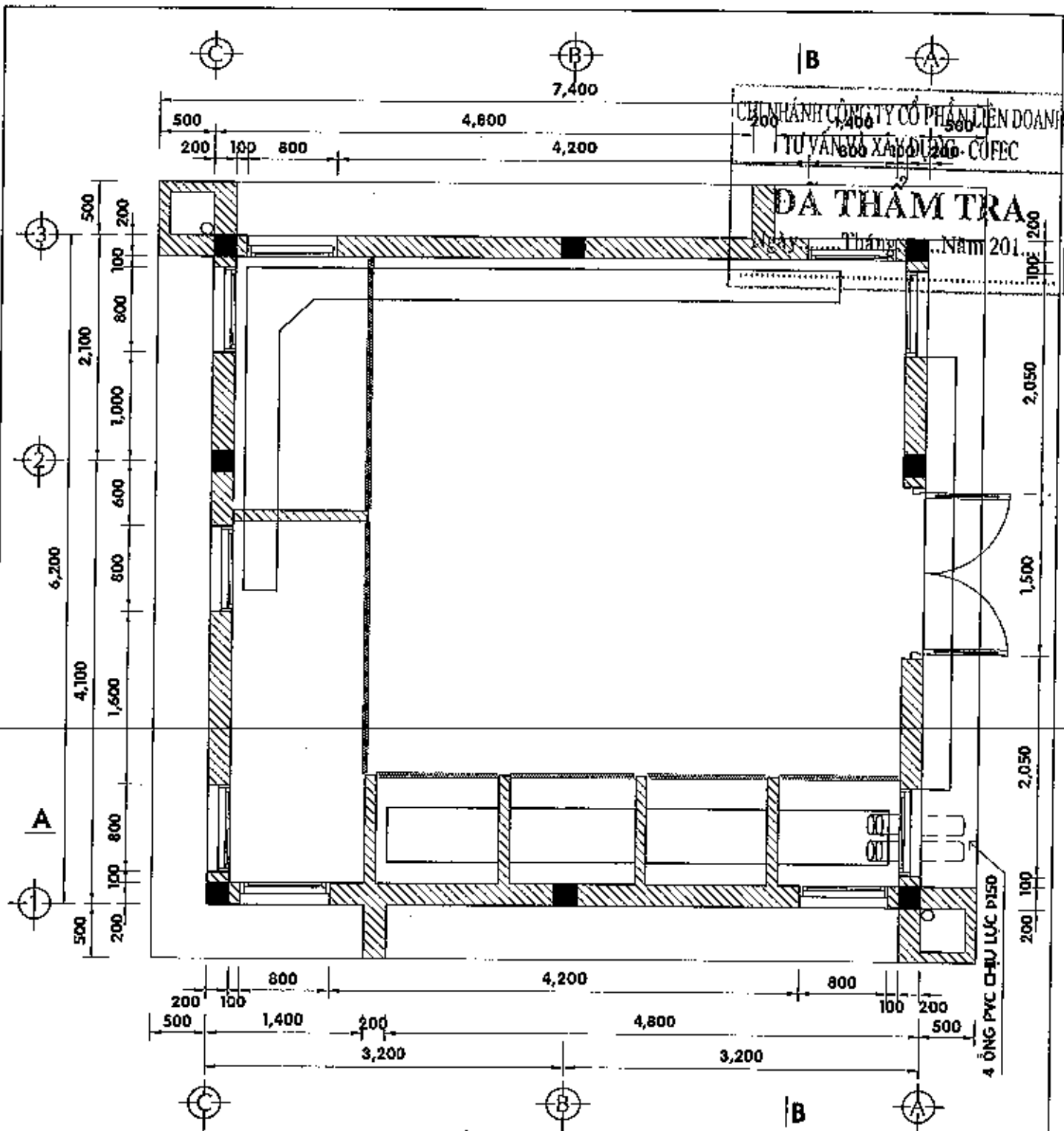
MẶT BẰNG TRẠM - TL 1/50
