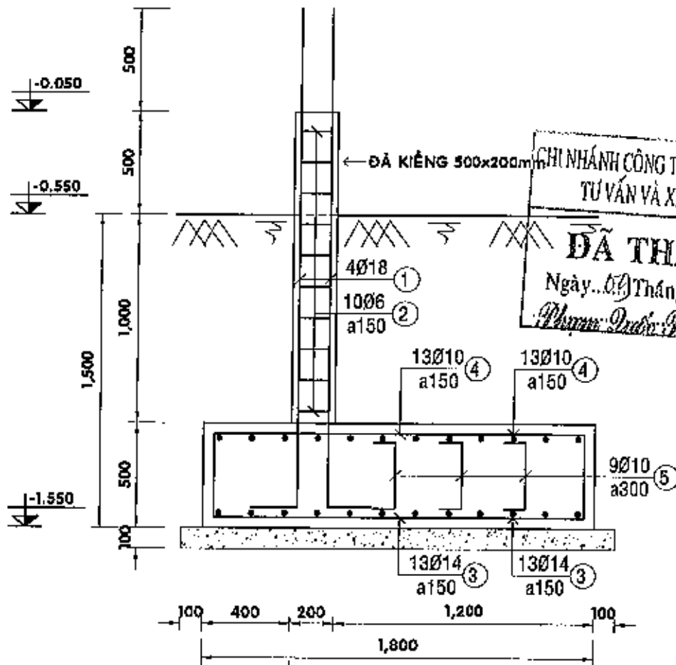
MẶT CẮT 7-7 - TL 1/25
