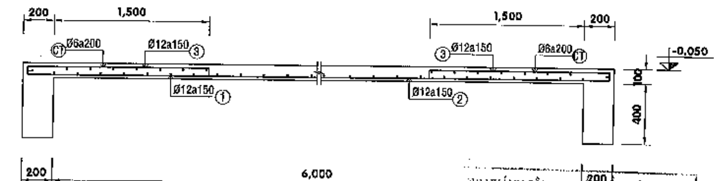
MẶT CẮT A-A - TL 1/25
