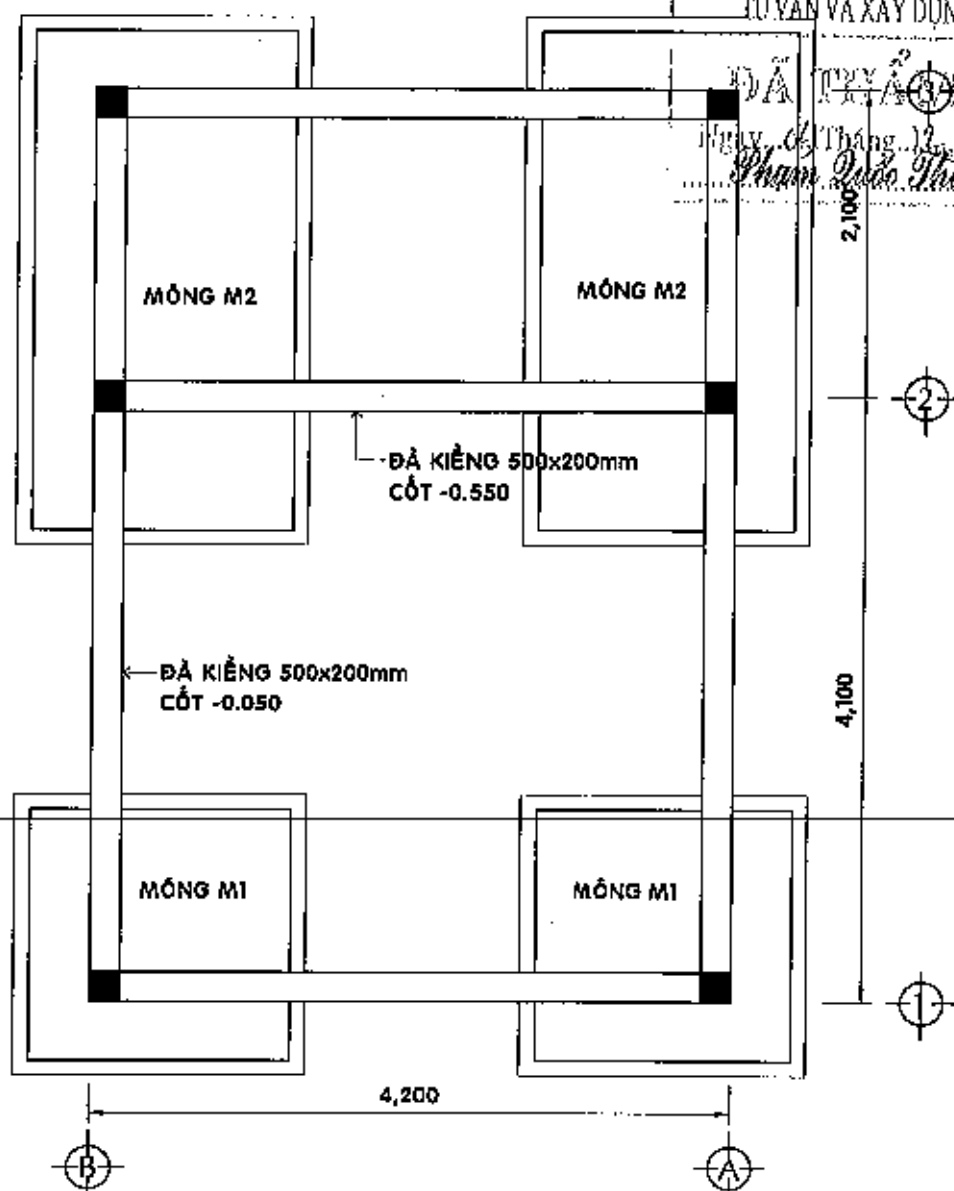
MẶT BẰNG BỐ TRÍ MÓNG - TL 1/50
