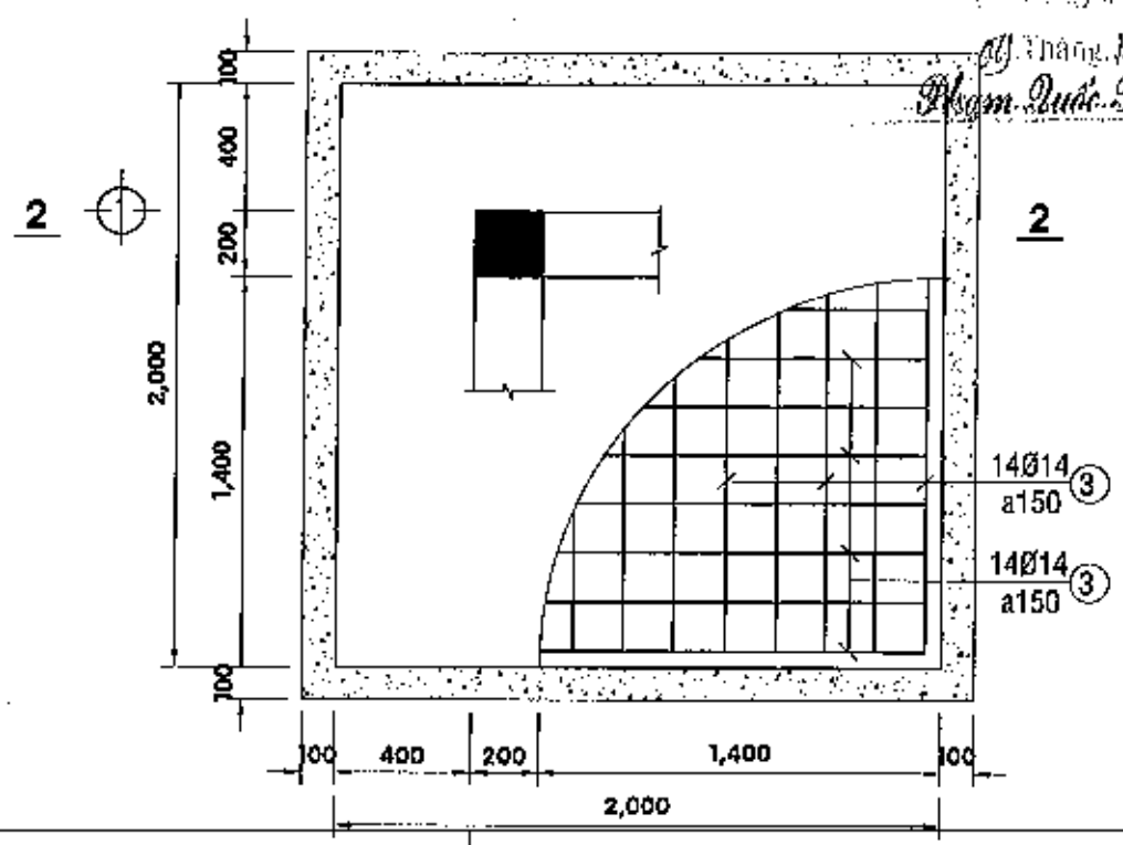
KẾT CẤU MÓNG M1 - TL 1/25 (LOẠI 2: KÍCH THƯỚC 2.0m x 2.0m)
