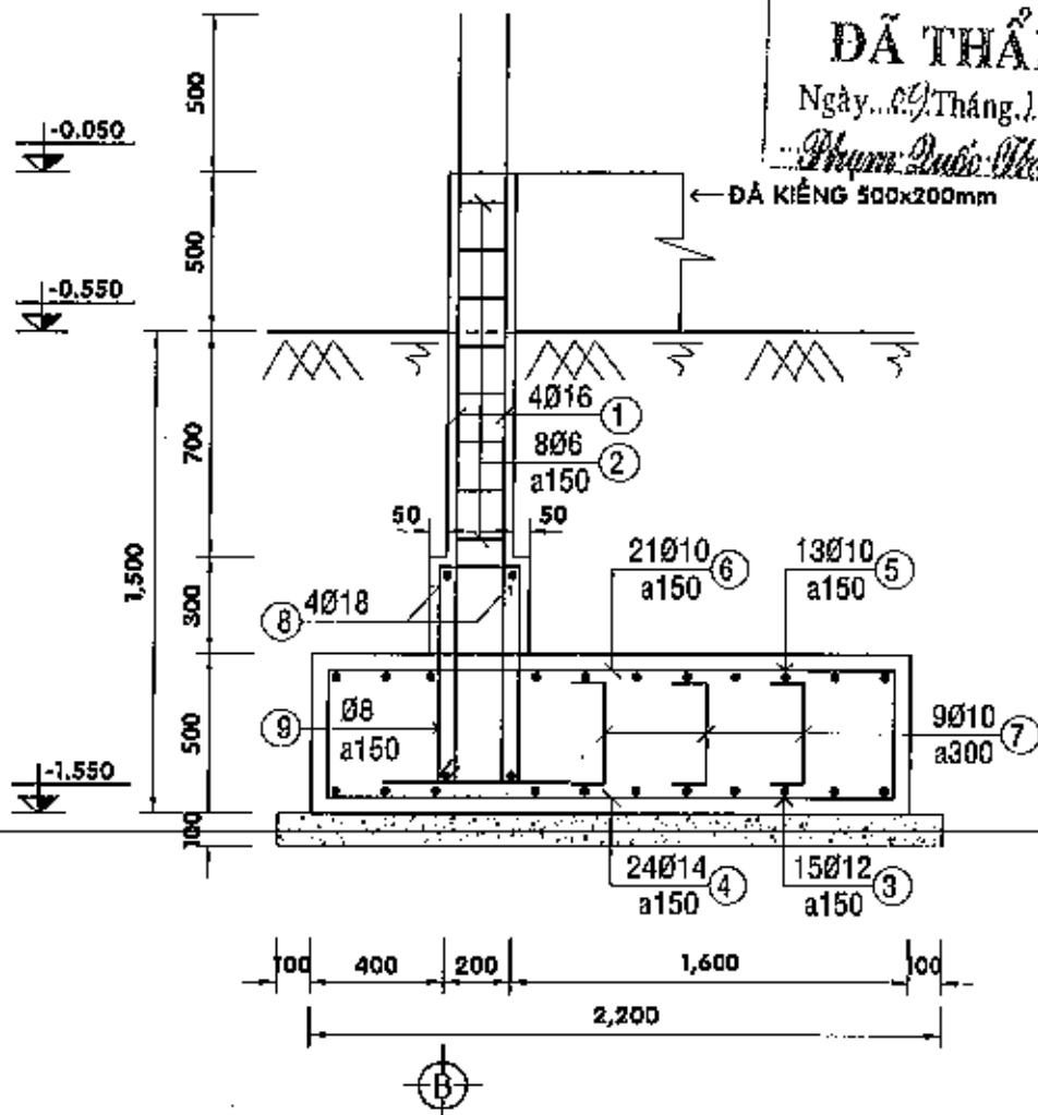
MẶT CẮT 5-5 - TL 1/25
