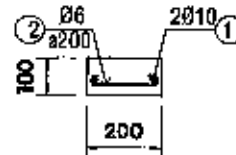
CỘT THÉP LANH TỜ THÔNG GIÓ - TL 1/20
