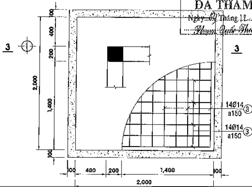
KẾT CẤU MÓNG M1 - TL 1/25 (LOẠI 3: KÍCH THƯỚC 2.0mx2.0m)
