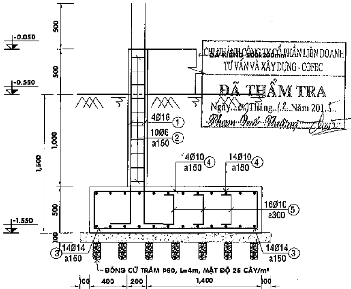
MẶT CẮT 3-3 - TL 1/25
