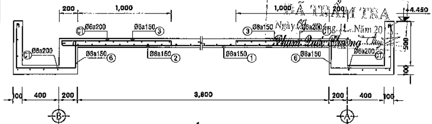
MẶT CẮT B-B - TL 1/25
