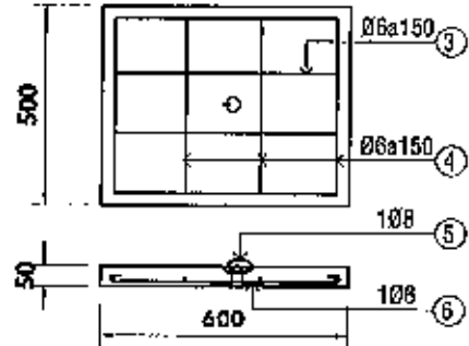
MƯƠNG TRUNG THỂ - TL 1/20
