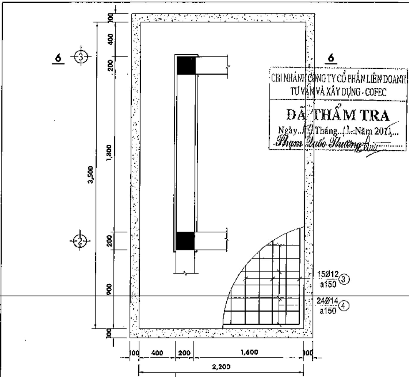
KẾT CẤU MÔNG M2 - TL 1/25 (LOẠI 3: KÍCH THƯỚC 3.5mx2.2m)
