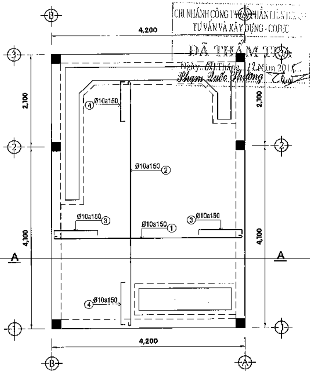
MẶT BẰNG THÉP SÀN TRỆT - TL 1/50
