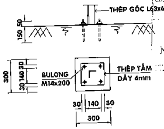
CHI TIẾT CHÂN ĐỀ - TL 1/25
