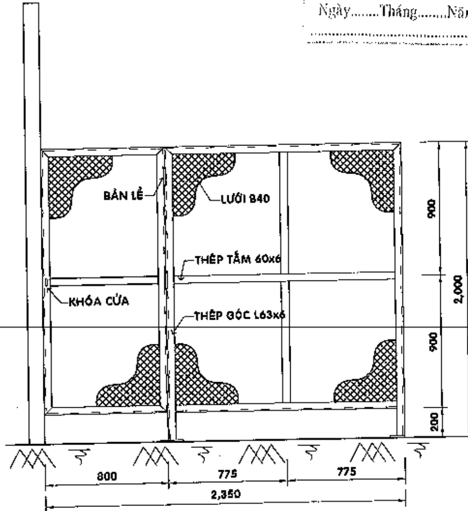
CHI TIẾT HÀNG RÀO LƯỚI B40 - TL 1/25
