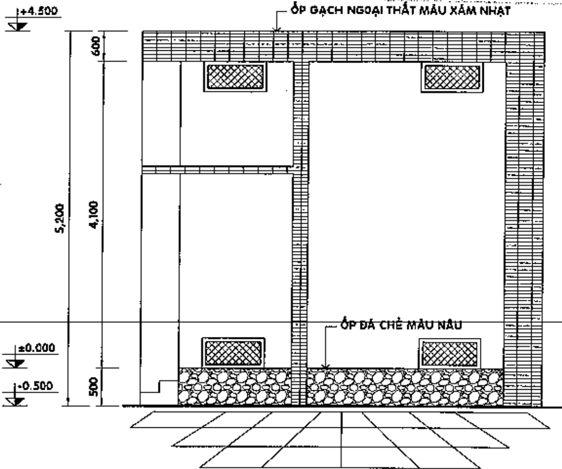
MẶT ĐỨNG TRỤC A-B - TL 1/50
