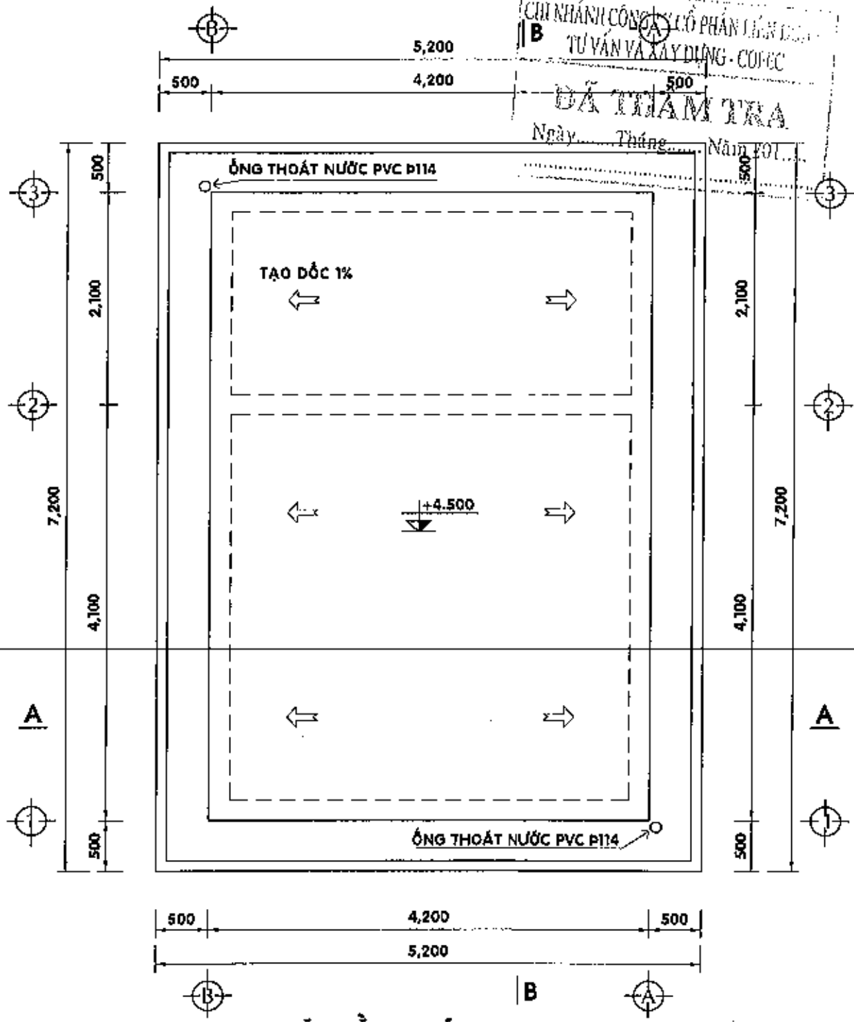
MẶT BẰNG MÁI - TL 1/50
