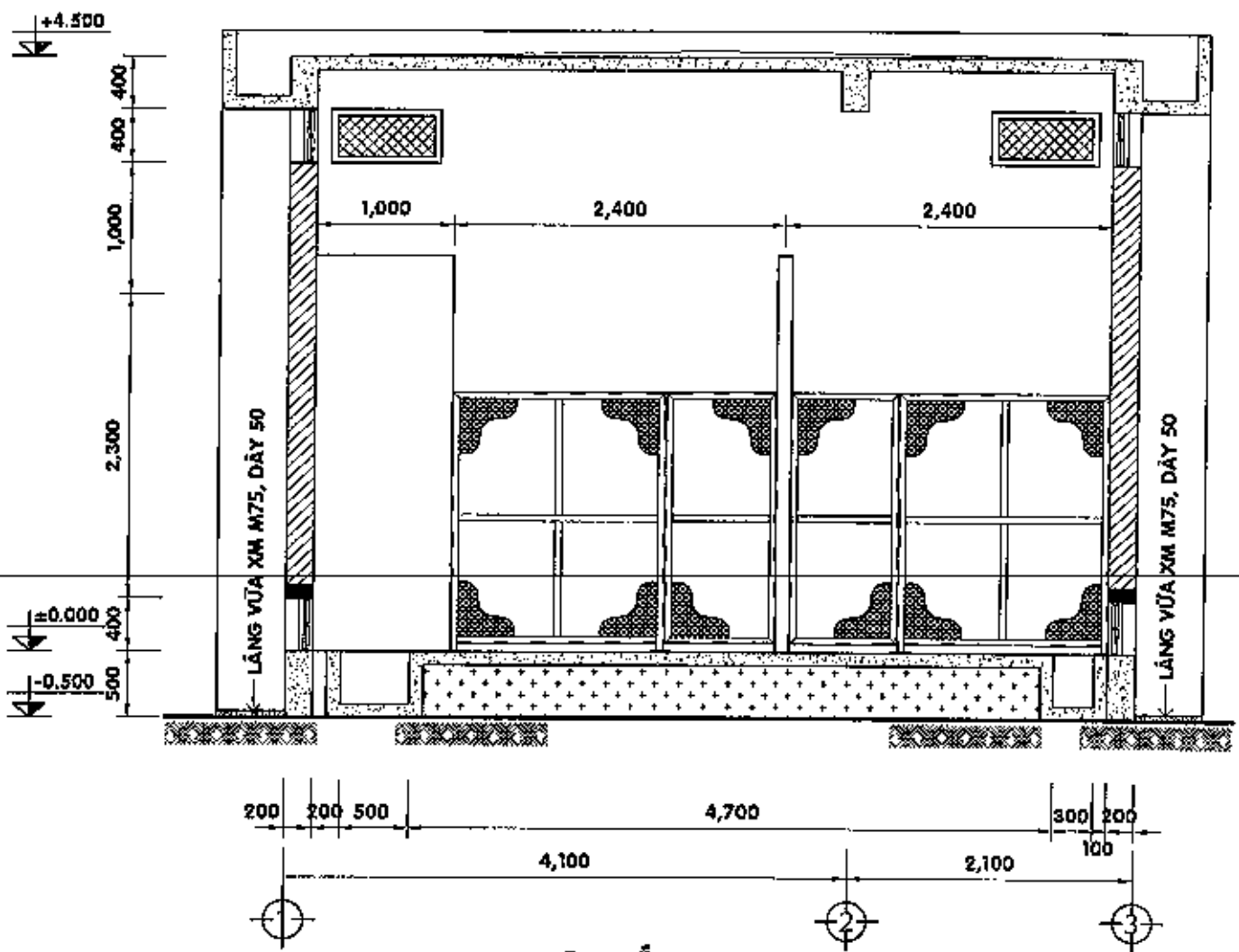
MẶT CẮT B-B - TL 1/50
