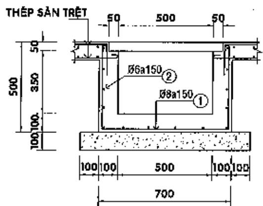
MƯƠNG TRUNG THỂ - TL 1/20
