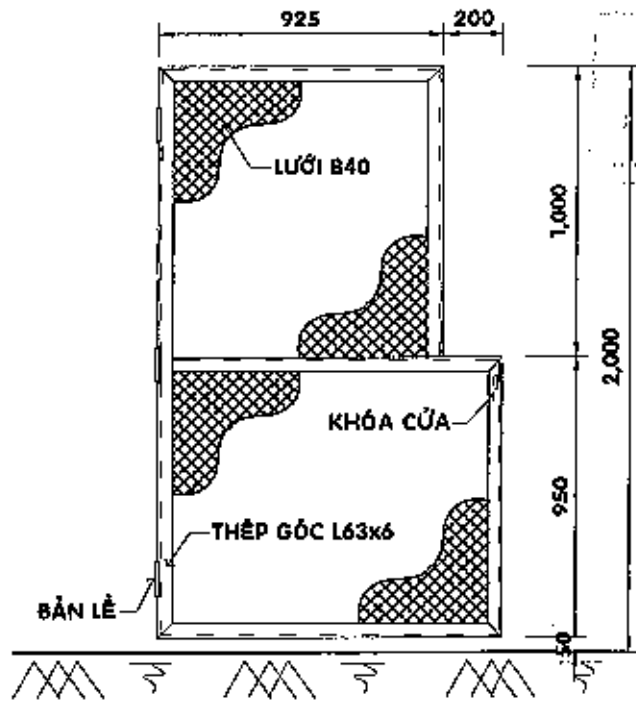
CHI TIẾT HÀNG RÀO LƯỚI B40 - TL 1/25
