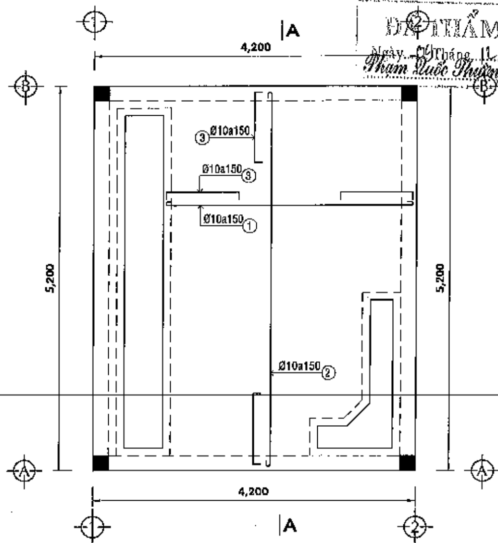
MẶT BẰNG THÉP SÀN TRỆT - TL 1/50
