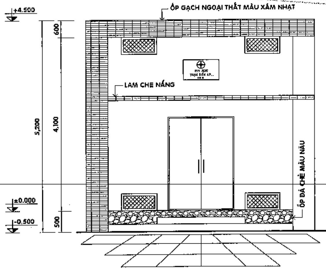
MẶT ĐỨNG TRỤC 1-2 - TL 1/50
