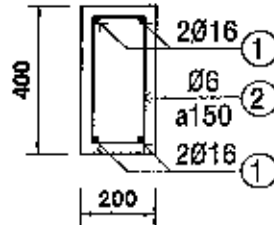
CỘT THÉP DẪM MẮI - TL 1/20
