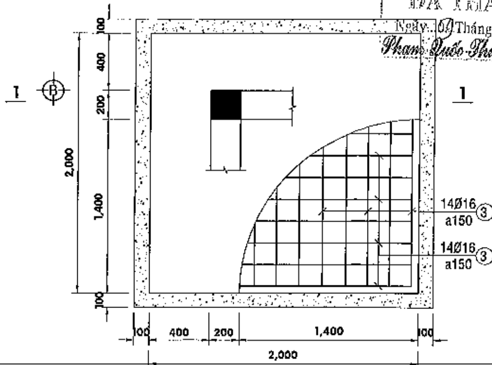
KẾT CẤU MÓNG M1 - TL 1/25 (LOẠI 1: KÍCH THƯỚC 2.0mx2.0m)
