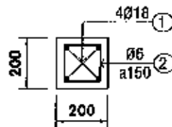
CỘT THÉP CỘT - TL 1/20
