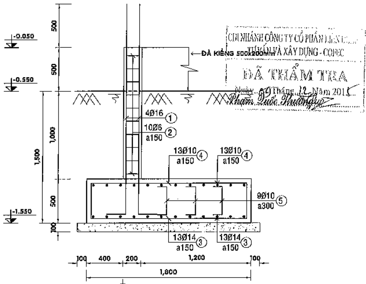
MẶT CẮT 1-1 - TỈ 1/25
