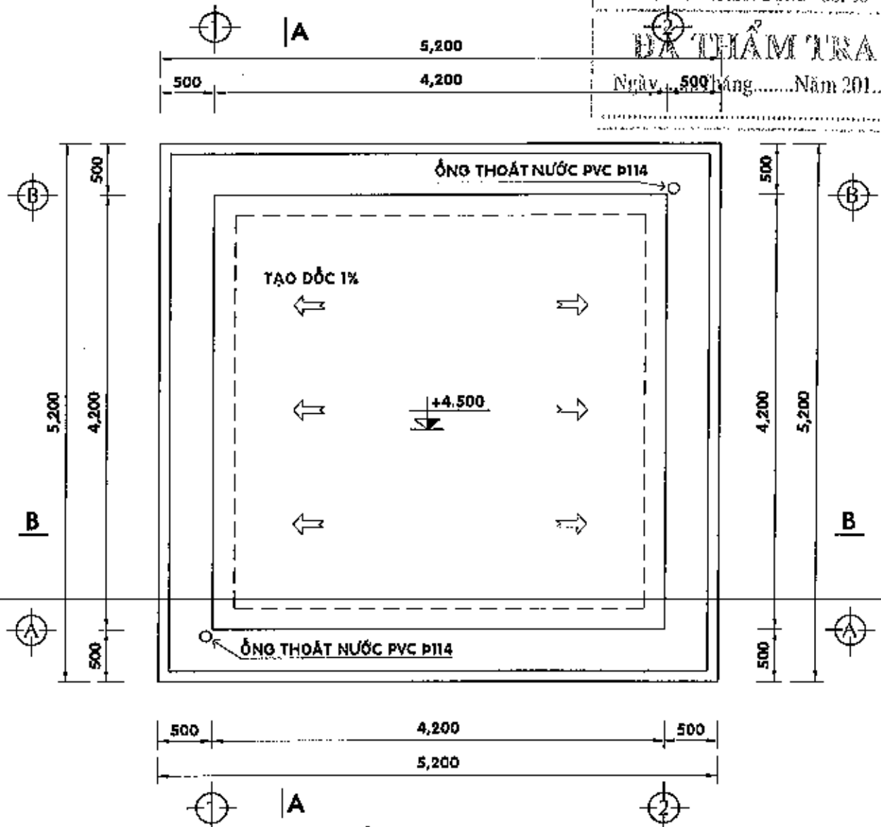
MẶT BẰNG MÁI - TL 1/50
