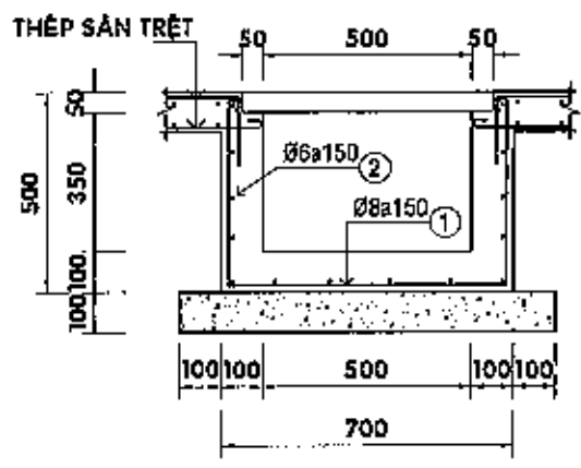
MƯƠNG TRUNG THỂ - TL 1/20
