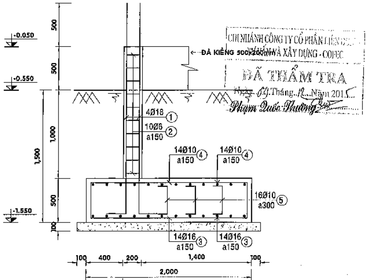
MẶT CẮT 1-1 - TL 1/25
