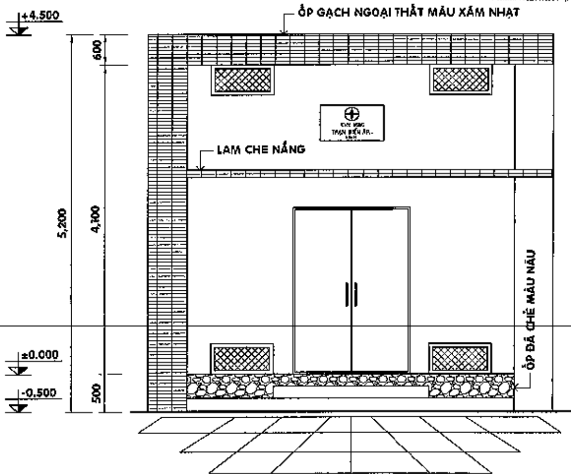
MẶT ĐŨNG TRỰC 1-2 - TL 1/50
