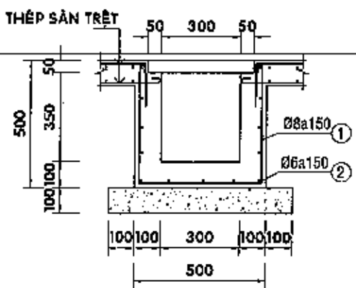
MƯƠNG HẠ THỂ - TL 1/20
