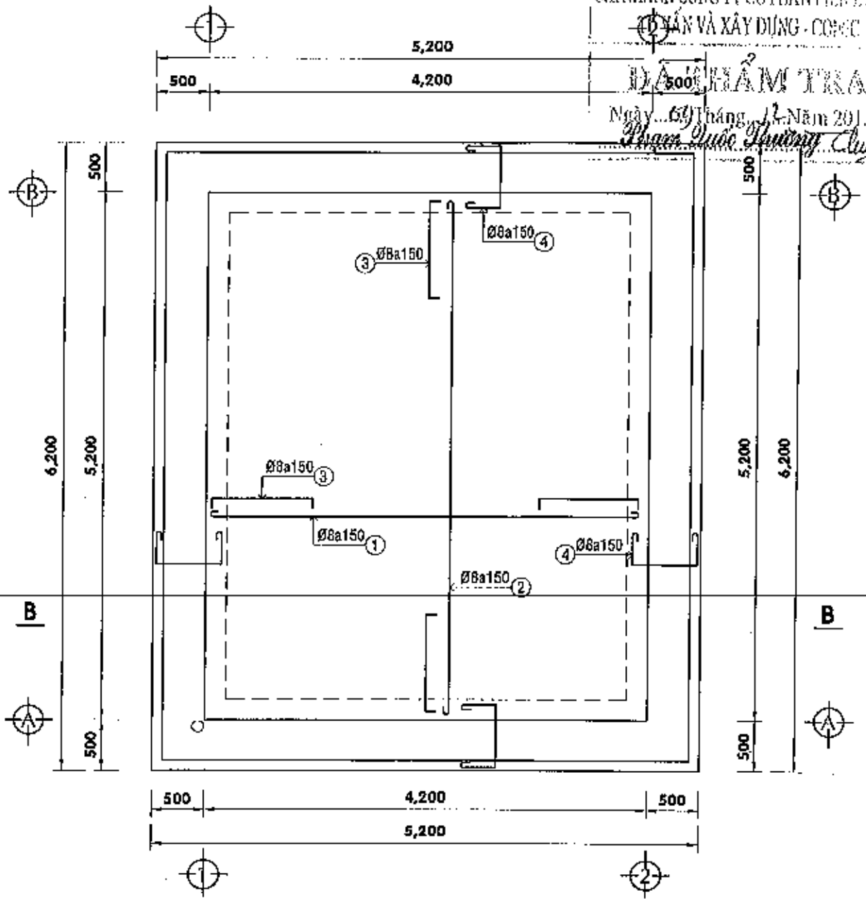
MẶT BẰNG THÉP SÀN MÁI - TL 1/50
