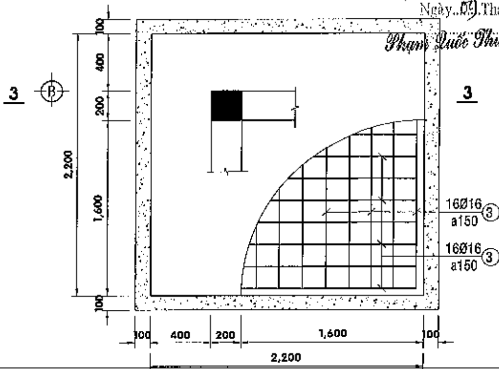
KẾT CẤU MÓNG M1 - TL 1/25 (LOẠI 3: KÍCH THƯỚC 2.2mx2.2m)
