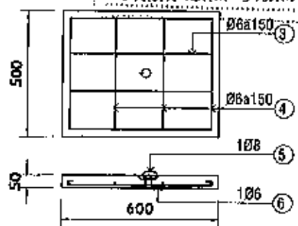
MƯƠNG TRUNG THỂ - TL 1/20
