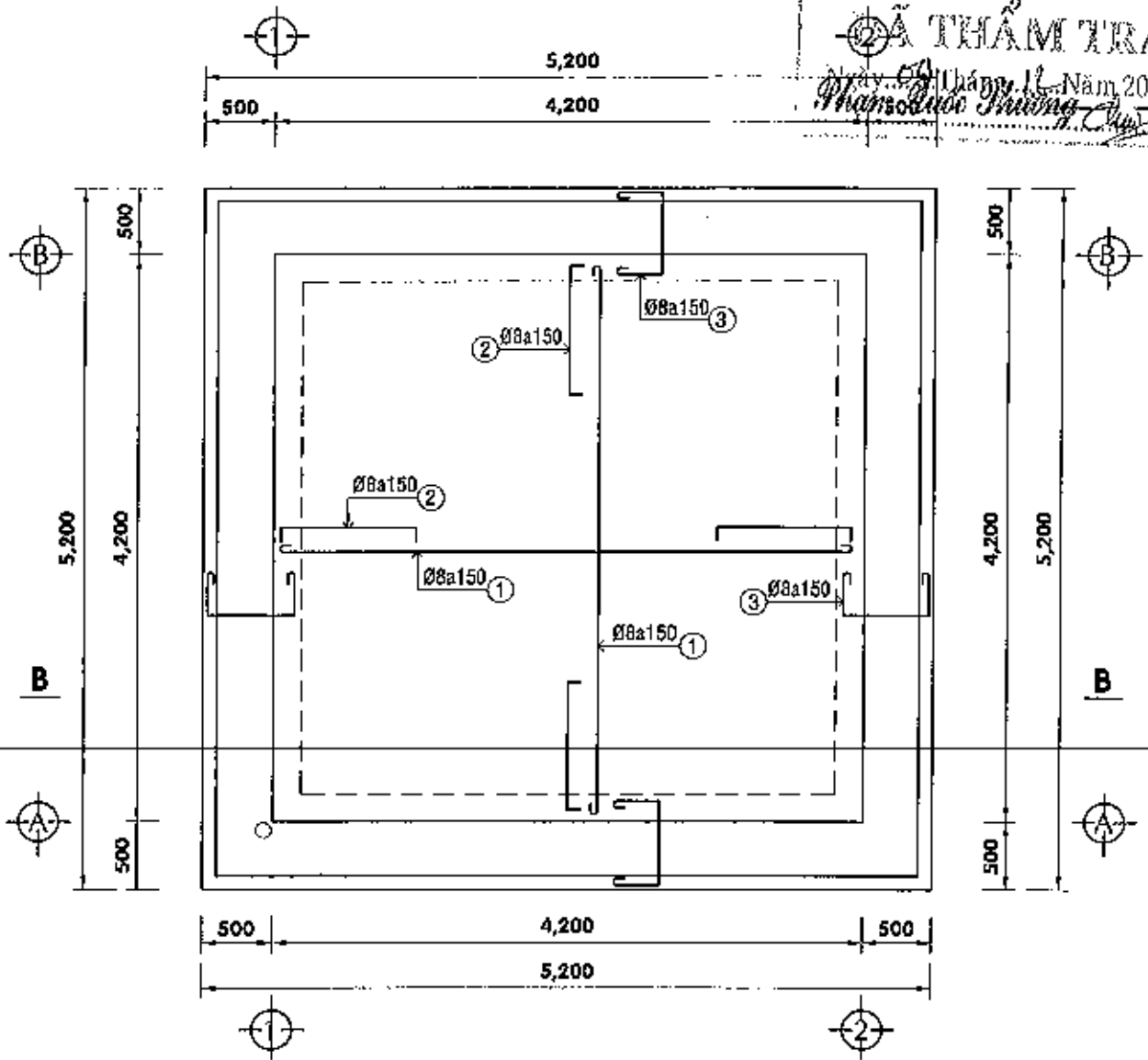
MẶT BẰNG THÉP SÀN MÁI - TL 1/50
