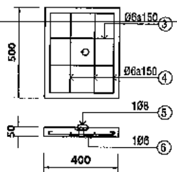
MƯƠNG HẠ THỂ - TL 1/20
