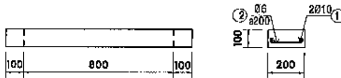
CỘT THÉP LANH TỜ THÔNG GIÓ - TL 1/20
