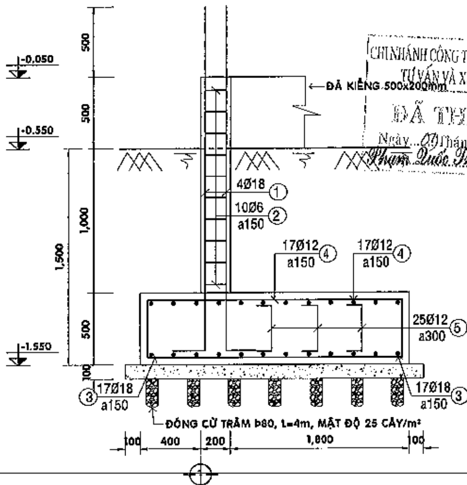
MẶT CẮT 3-3 - TL 1/25
