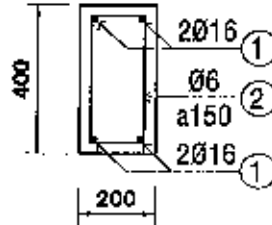
CỘT THÉP DẦM MÁI - TL 1/20
