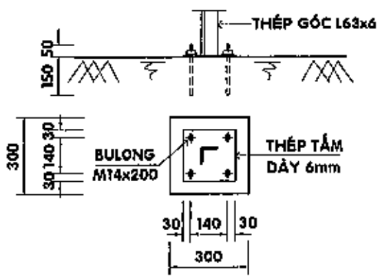
CHI TIẾT CHÂN ĐỂ - TL 1/20
