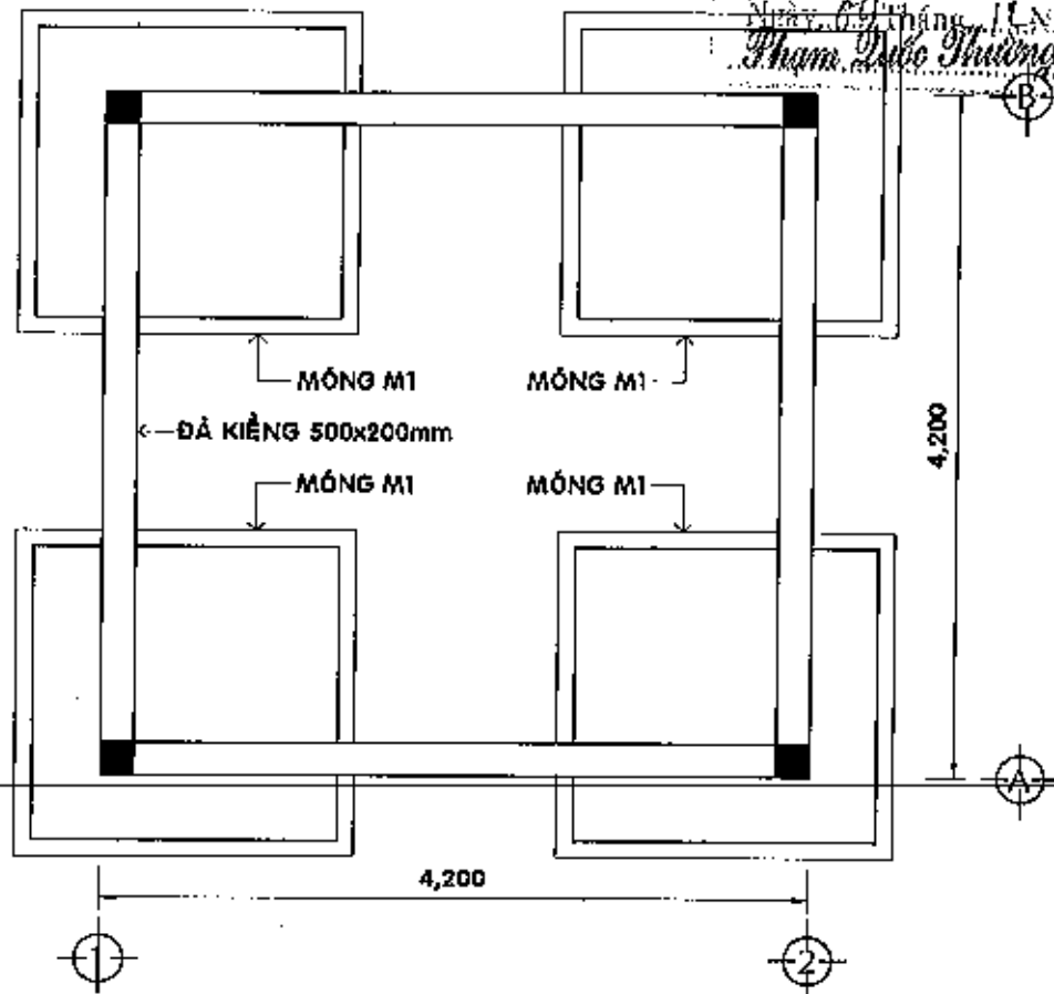
MẶT BẰNG BỐ TRÍ MÓNG - TL 1/50
