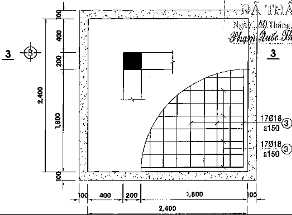
KẾT CẤU MÓNG M1 - TL 1/25 (LOẠI 3: KÍCH THƯỚC 2.4m x 2.4m)
