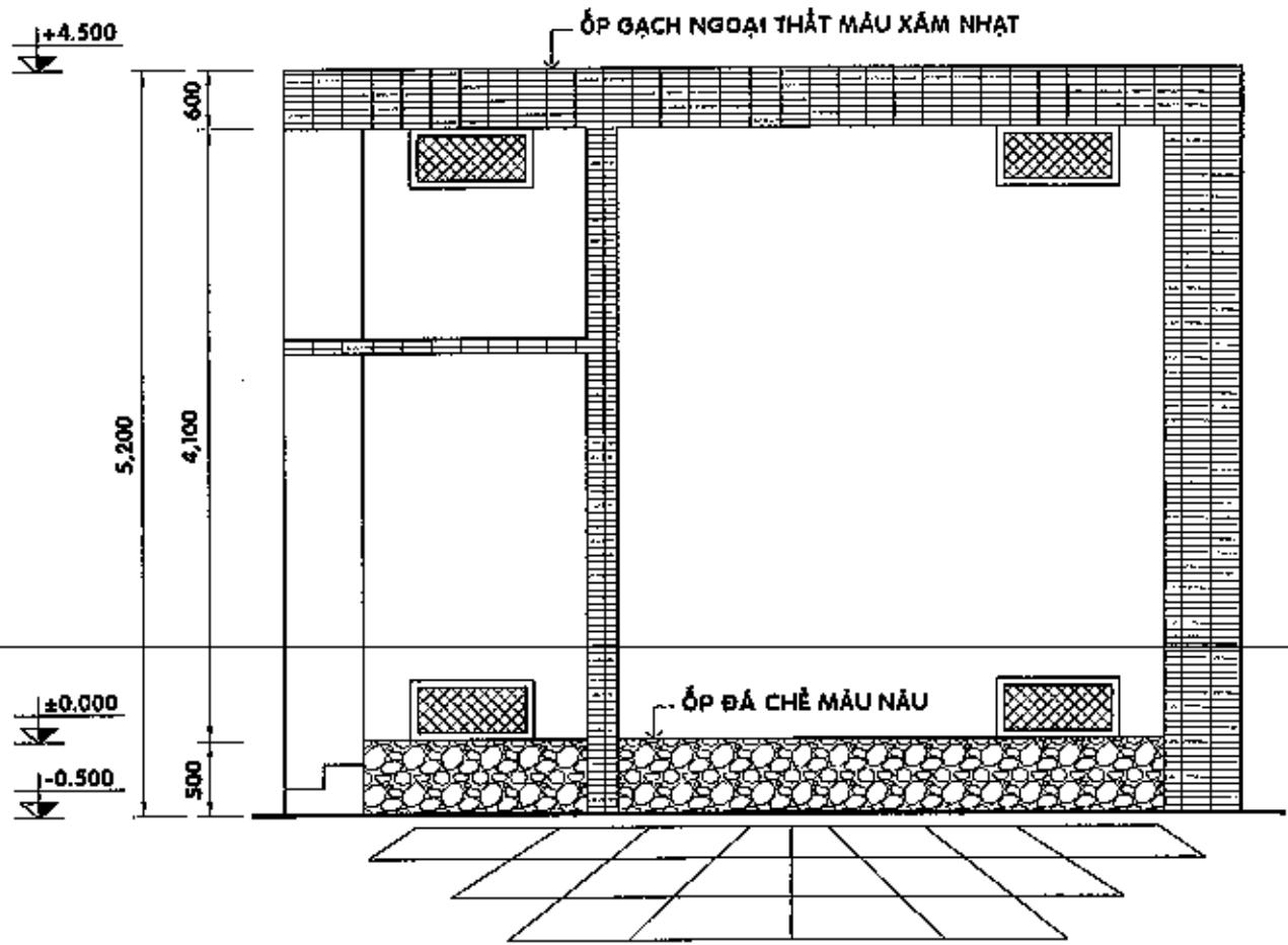
MẶT ĐỨNG TRỤC A-B - TL 1/50
