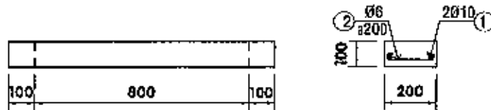
CỘT THÉP LANH TỔ THÔNG GIÓ - TL 1/20
