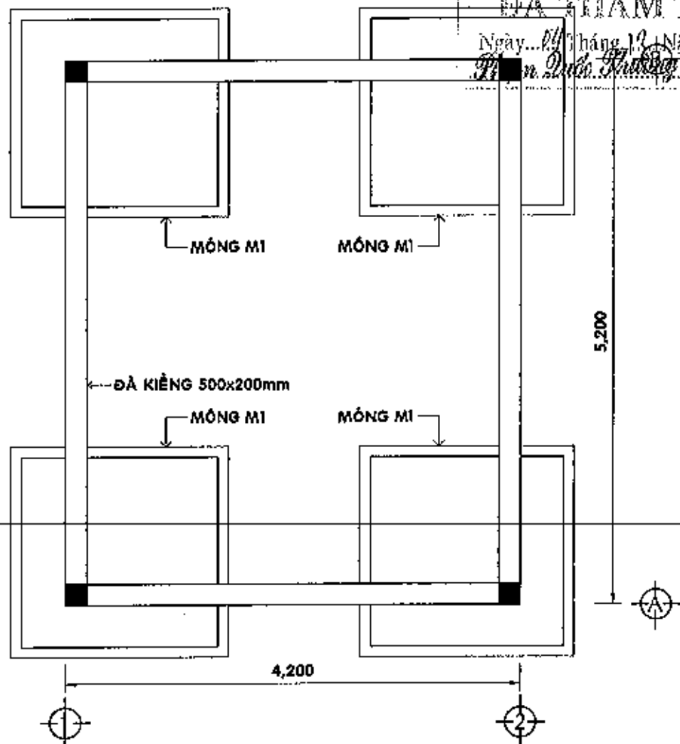
MẶT BẰNG BỐ TRÍ MÓNG - TL 1/50
