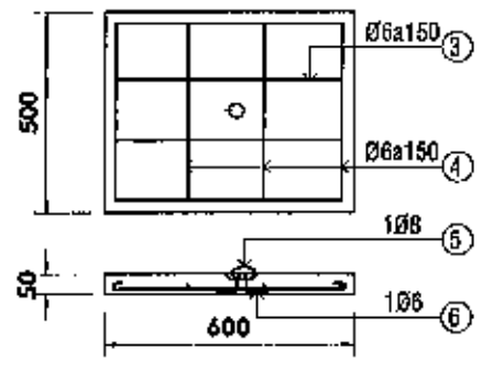
MƯƠNG TRUNG THỂ - TL 1/20
